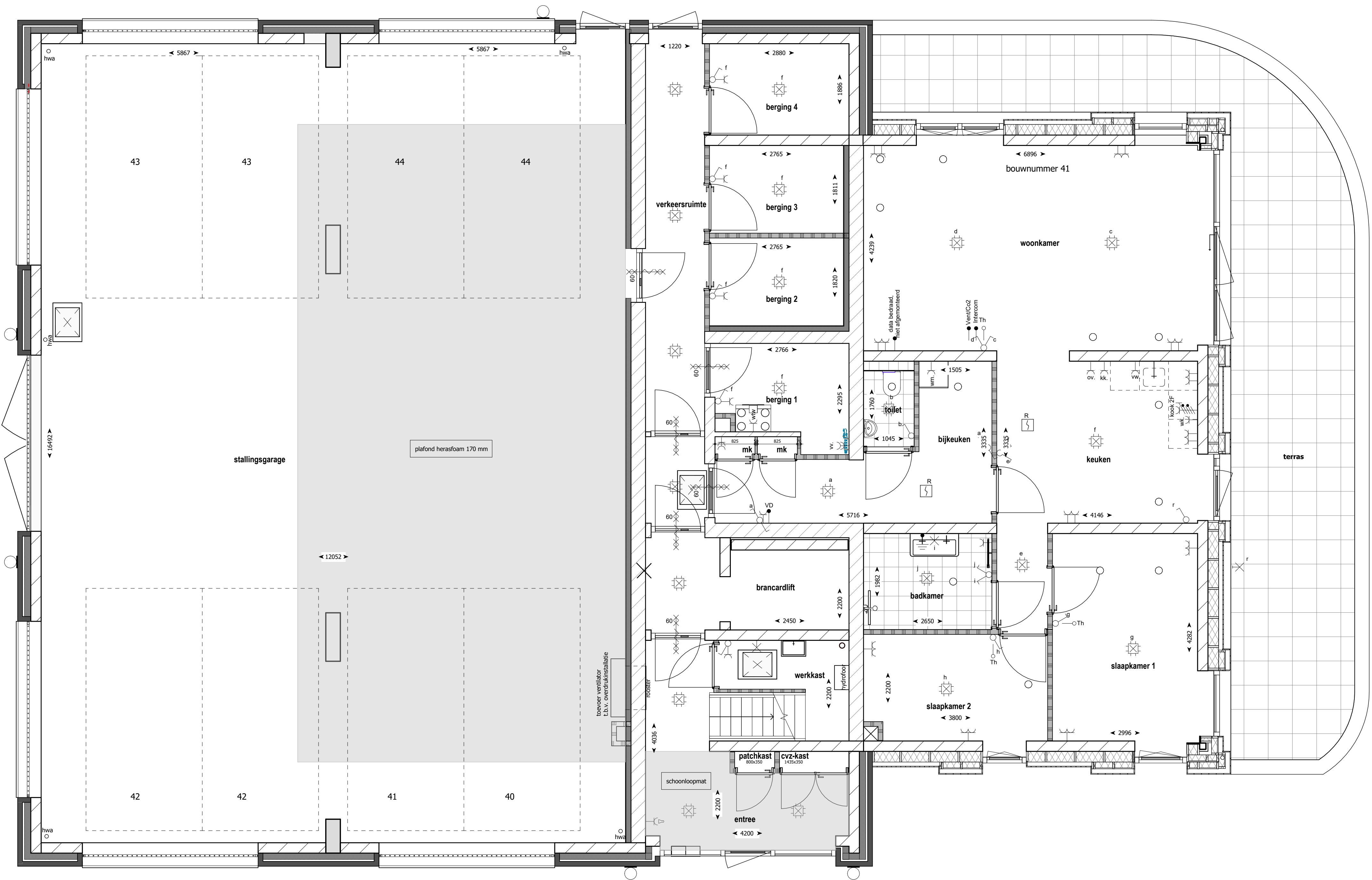
Begane grond 1 : 50
