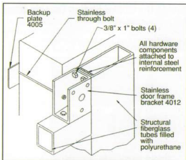
Horizontal Door Frame Diagram
