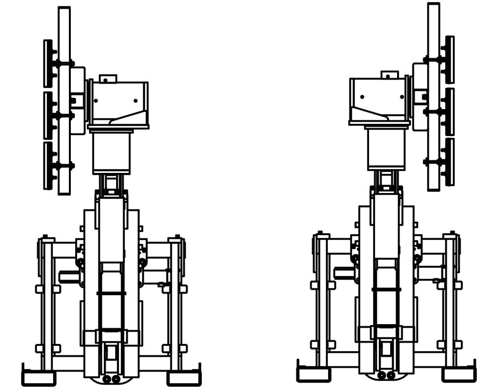
Seitliche Kippbarkeit: 180°
