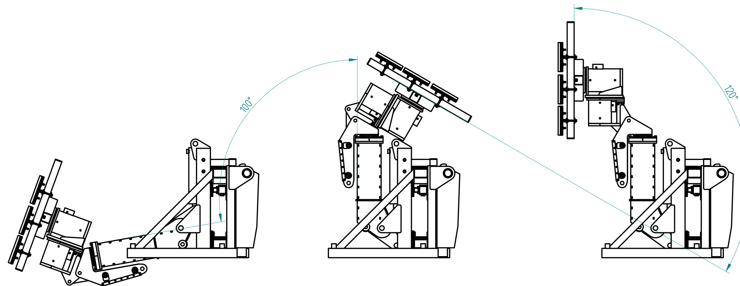
Schwenkbarkeit Ausleger: 100°
