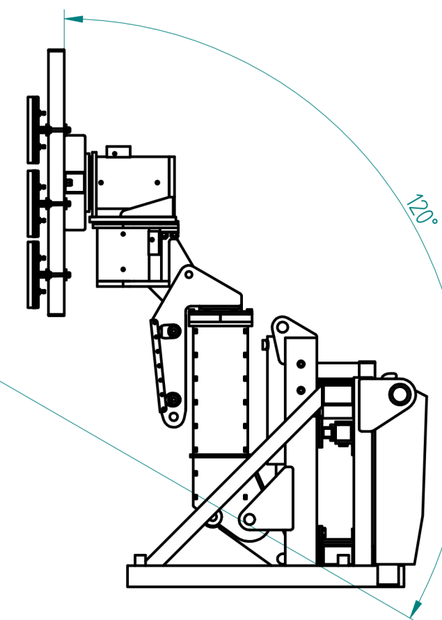
Schwenkbarkeit Saugerbrücke: 120°
