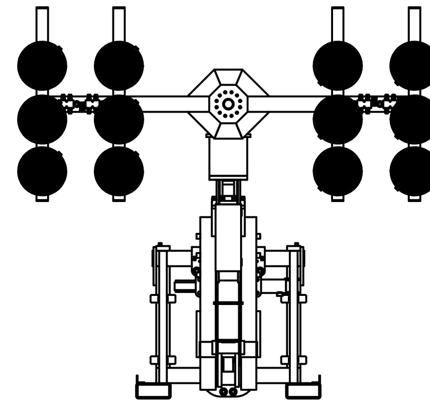
Drehbarkeit Saugerbrücke: 360°
