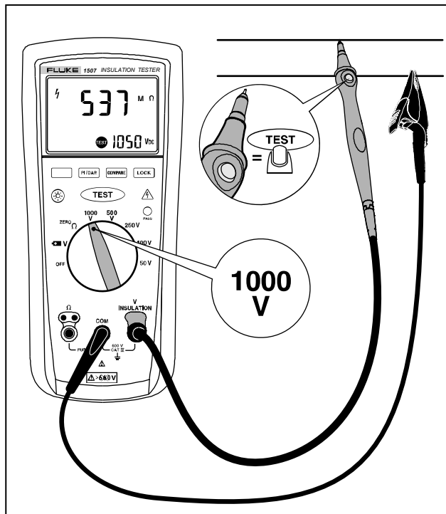
그림7. 절연 테스트
