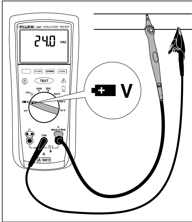
그림5. 전압 측정
