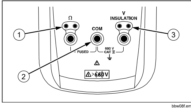
그림 4. 입력 단자
