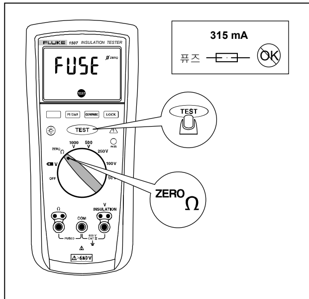
그림 10. 퓨즈 테스트
