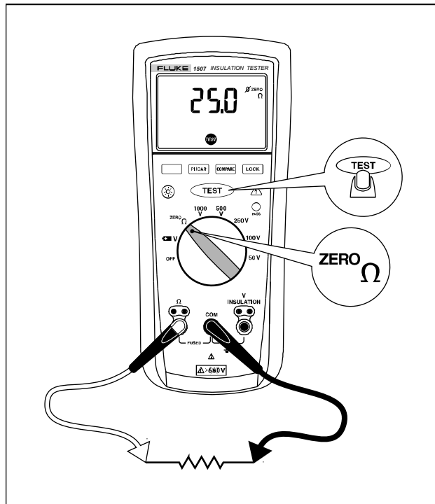
그림6. 저항 측정
