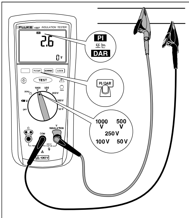
그림 8. 극성화 인텍스 및 유전체 흡수율 측정
