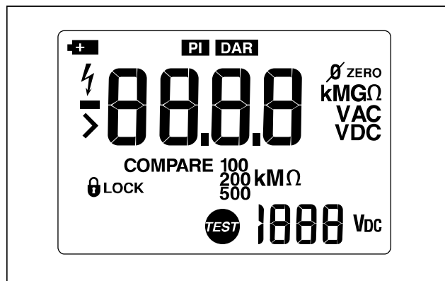
그림3. 디스플레이 표시
