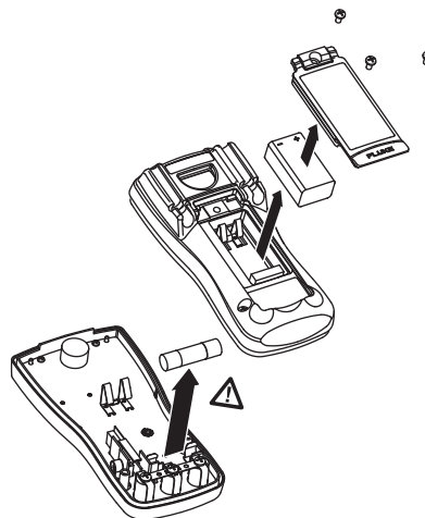
그림 2. 분해
