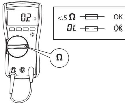
그림 1. 퓨즈 테스트
