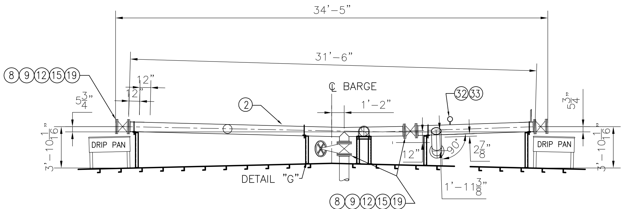
SECTION F-F SCALE:- N.T.S.
