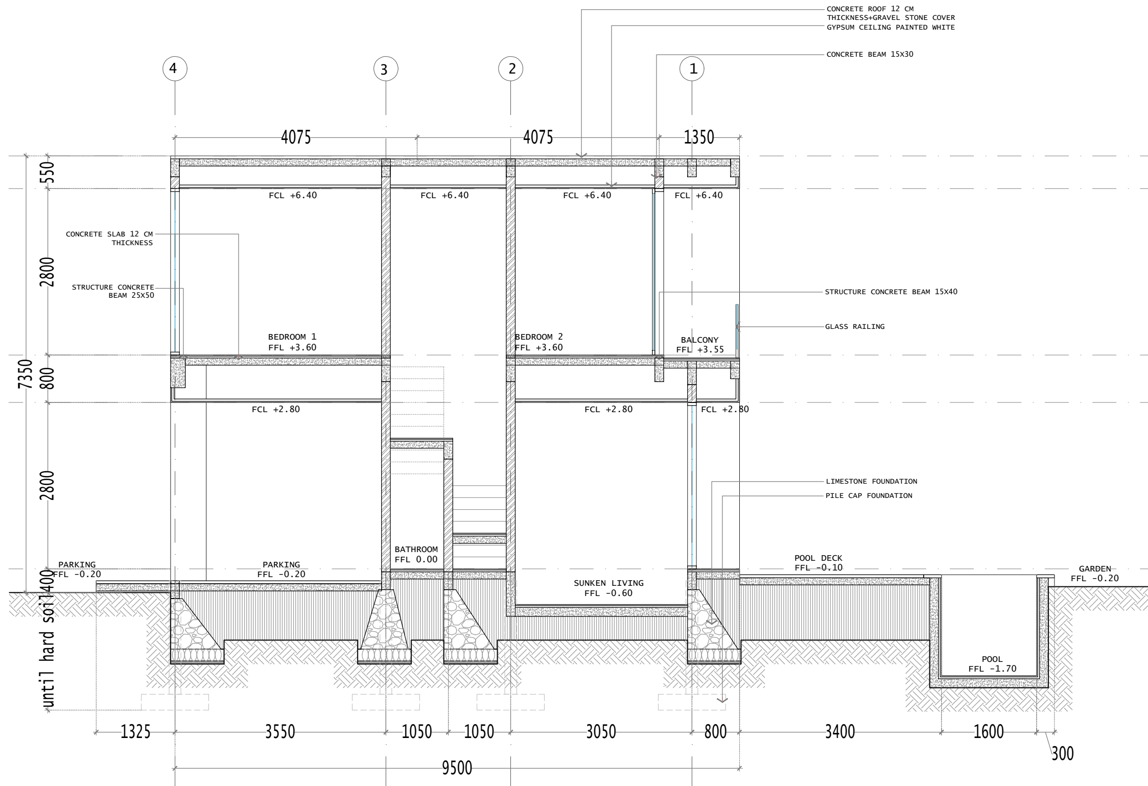
SECTION A-A SCALE 1 : 75
