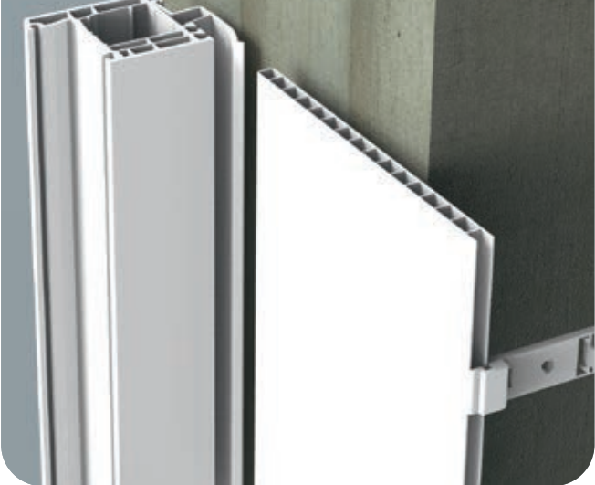
Držite ploču i jezičak zajedno na zidu i umetnite ih u prihvatni profil.
