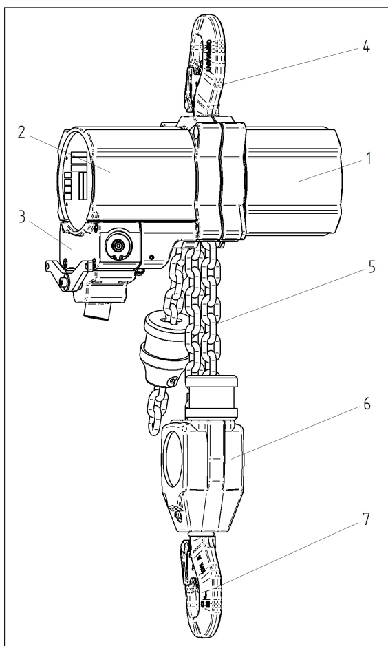
Figuur 3: Baugruppenübersicht
