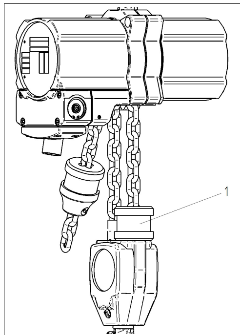
Figuur 6: Hefbegrenzer
