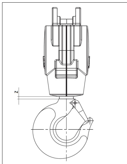
Figuur 18: Toelaatbare axiale speling
