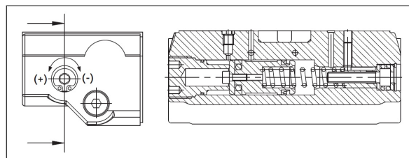
Figuur 14: Overbelastingsbeveiliging instellen
