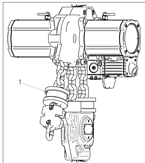
Abbildung 7: Senkbegrenzer
