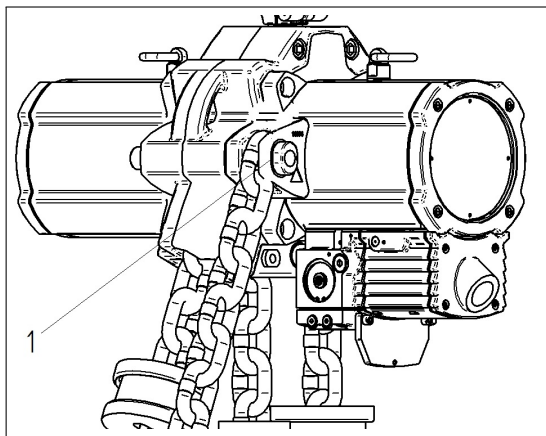
Abbildung 8: Leerstrangbefestigung
