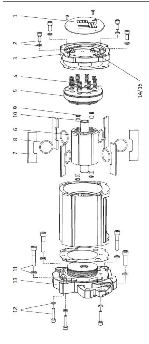
Abbildung 13: Hubmotor
