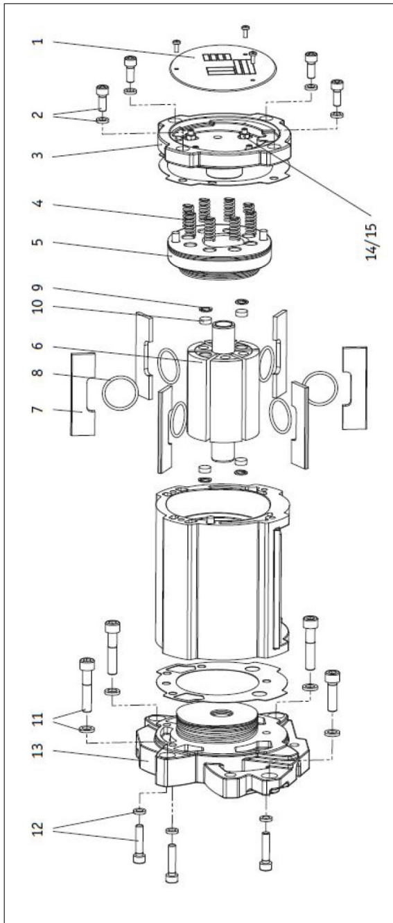
Abbildung 19: Hubmotor
