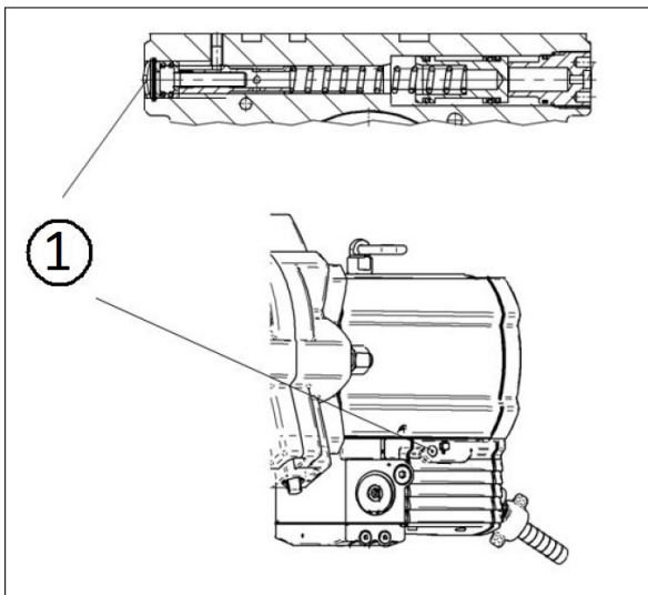
Abbildung 14: Überlastsicherung einstellen
