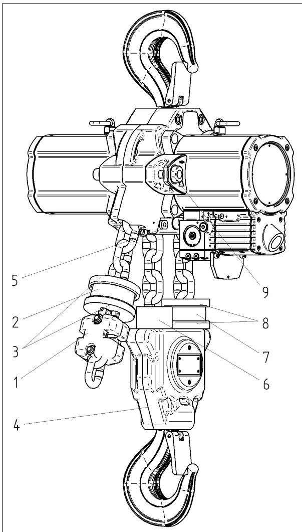
Abbildung 21: Kette austauschen
