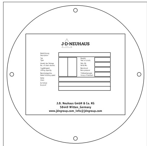
Abbildung 2: Typenschild PROFi 30 TI
