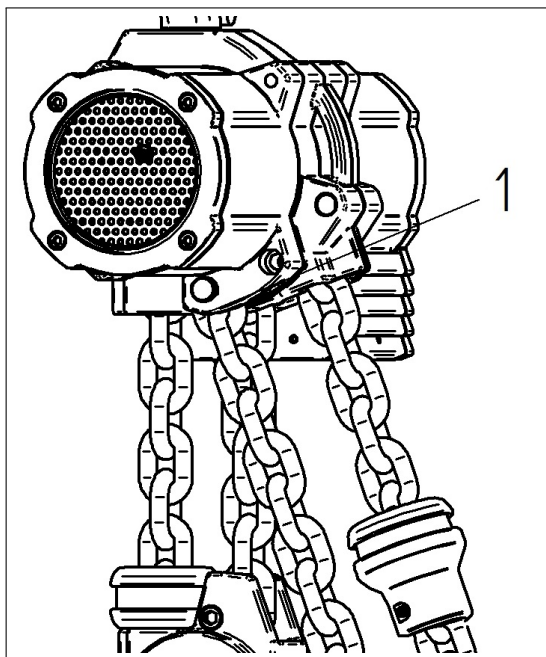
Figuur 8: Bevestiging lege strengen
