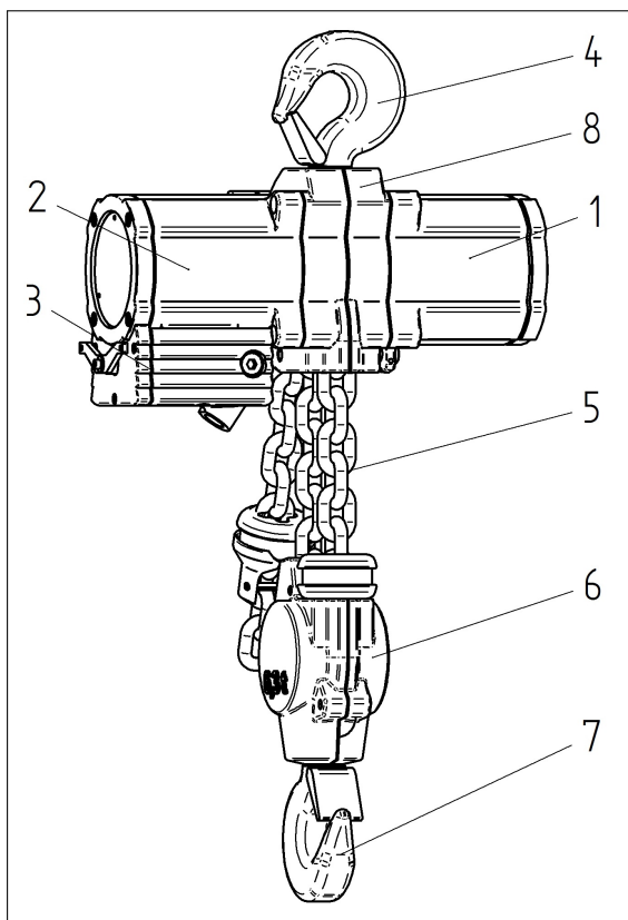
Figuur 3: Baugruppenübersicht
