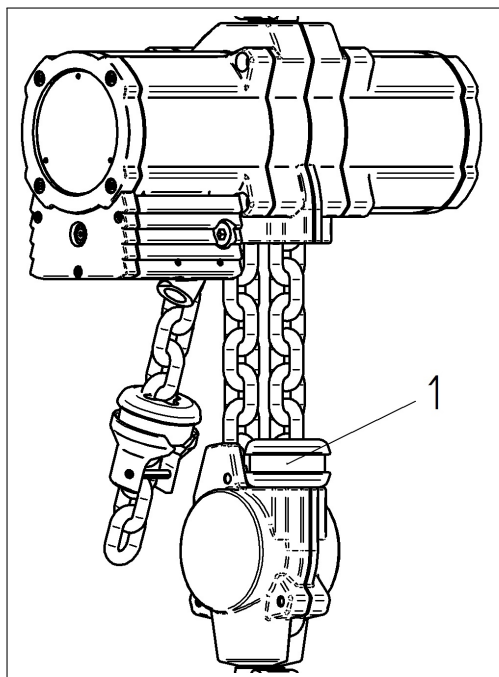
Figuur 6: Hefbegrenzer
