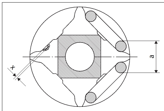
Figuur 15: Viertandig kettingwiel
