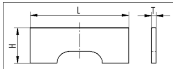
Figuur 19: Lamellen
