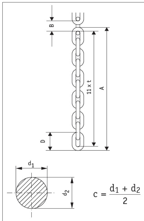
Figuur 14: Testmaten van de ketting
