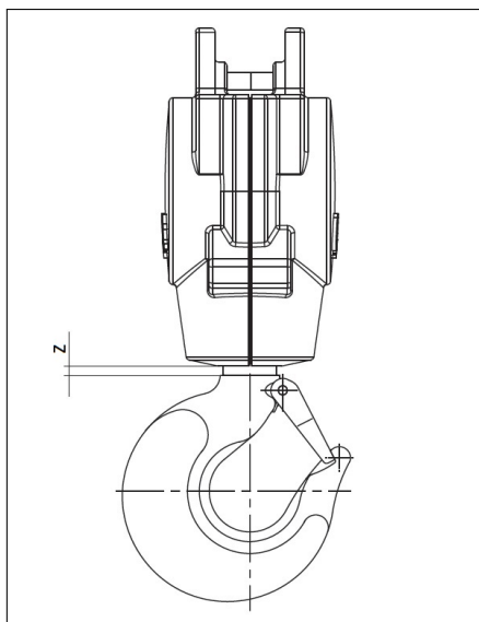
Figuur 17: Toelaatbare axiale speling
