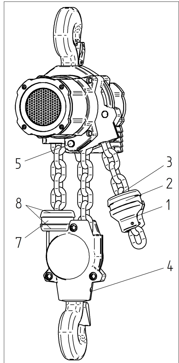
Figuur 20: Ketting vervangen
