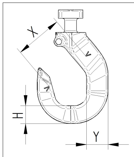
Figuur 16: Testmaten van de lasthaak (draaghaak)
