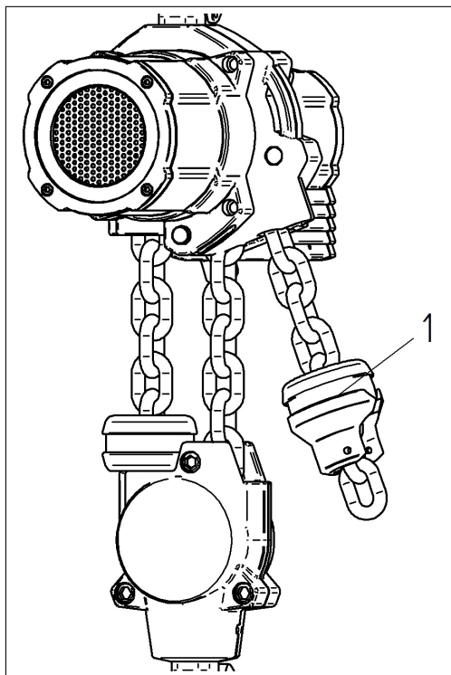
Figuur 7: Neerlaatbegrenzer
