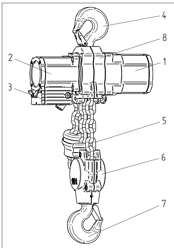
Figuur 3: Baugruppenübersicht
