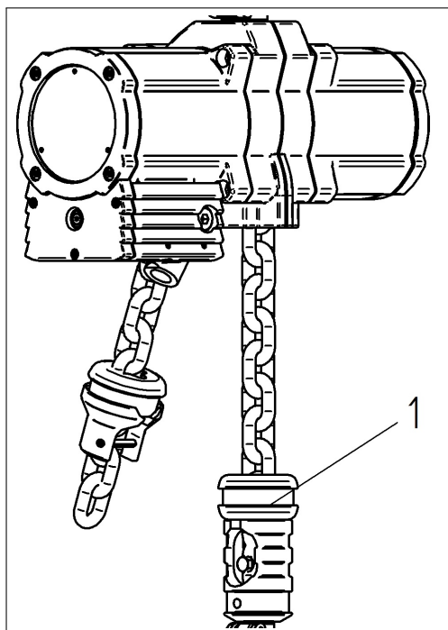
Figura 6: Limitador de elevación
