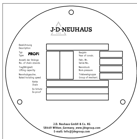
Figura 2: Placa de características PROFI 3 TI
