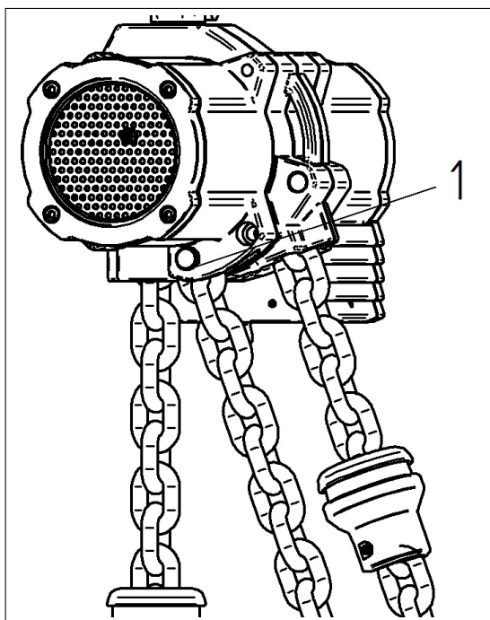
Figura 8: Fijación del ramal de retorno
