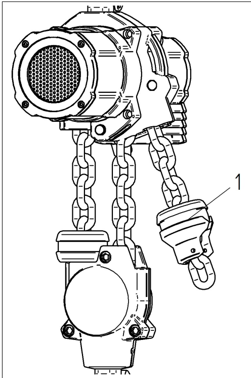
Figura 7: Limitador de descenso
