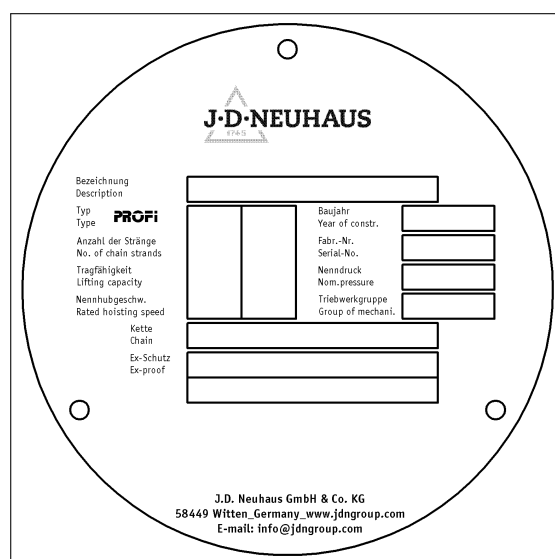
Figura 2: Placa de características PROFI 10 TI
