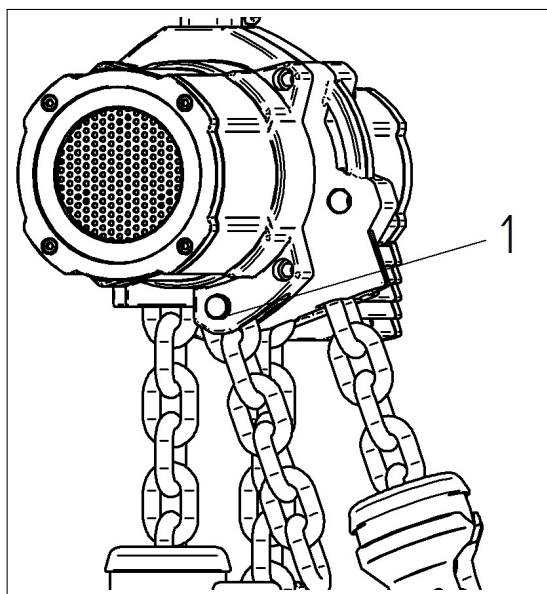
Figura 8: Fijación del ramal de retorno
