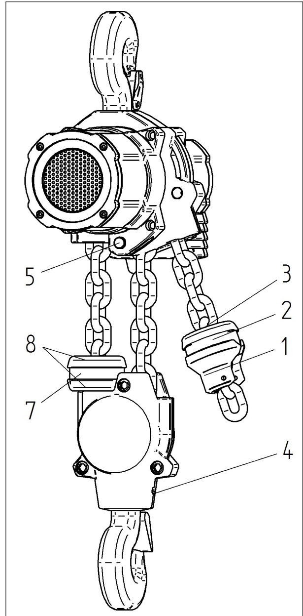
Figura 21: Cambio de cadena
