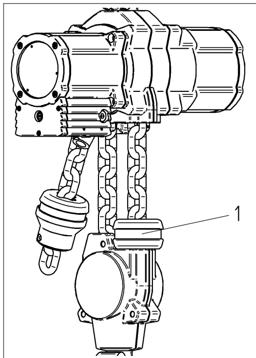
Figura 6: Limitador de elevación
