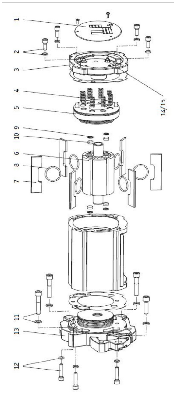
Figura 19: Motor de elevación
