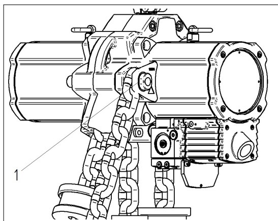
Figura 8: Fijación del ramal de retorno
