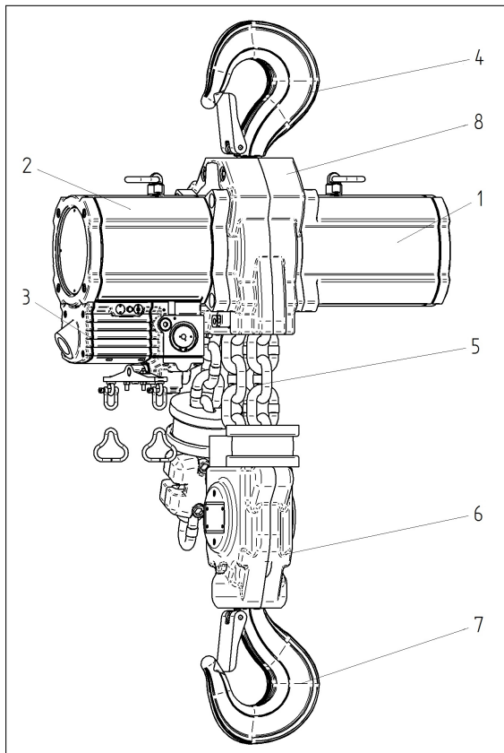
Figura 3: Relación de grupos constructivos
