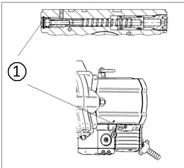
Figura 14: Ajuste del limitador de carga
