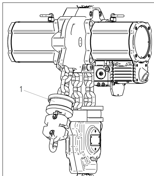
Figura 7: Limitador de descenso
