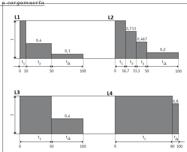
Figura 12: Esquema de conjuntos de cargas
