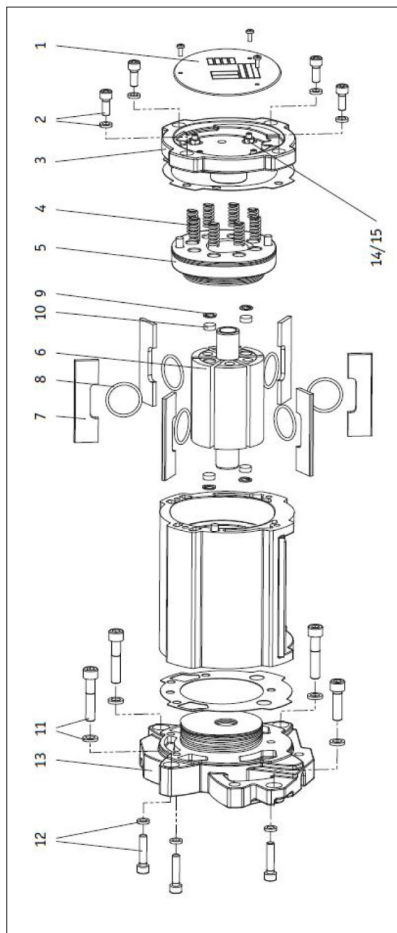
Figura 13: Motor de elevación
