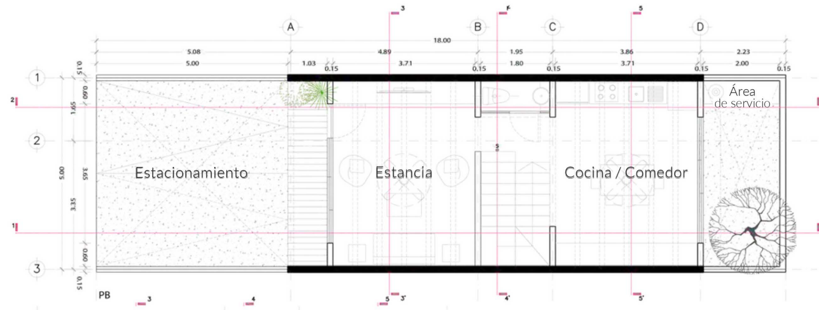
Planta baja
