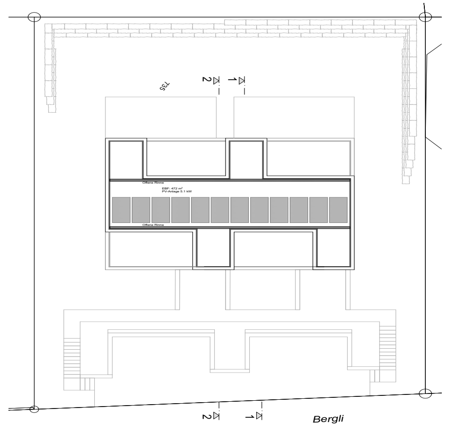
Dachaufsicht
