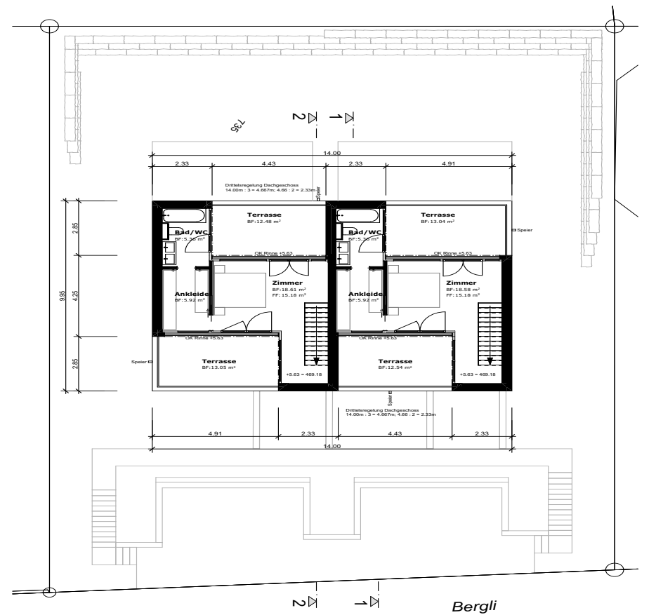
Dachgeschoss
