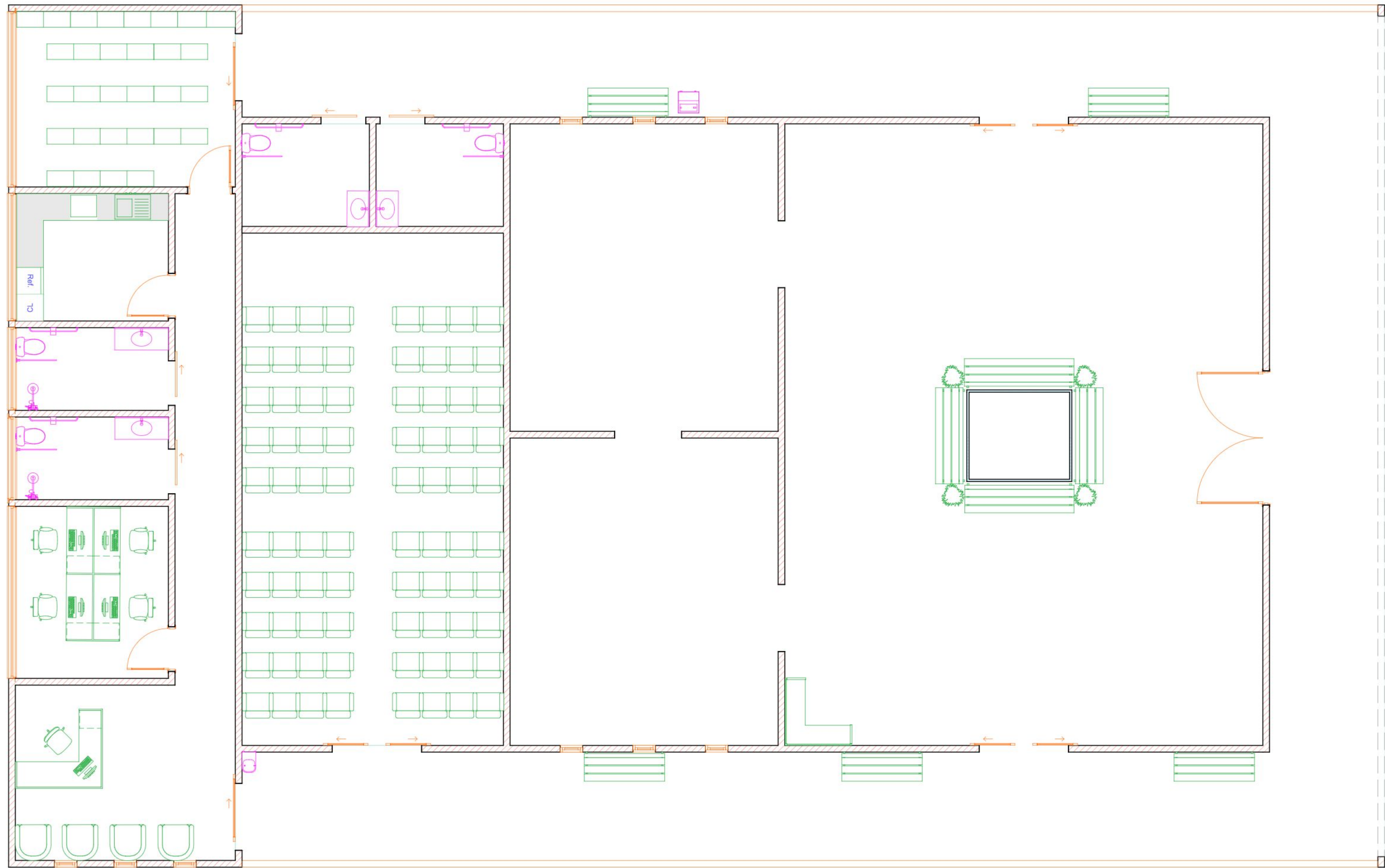
1 PLANTA DE LAYOUT Escala: 1:75
