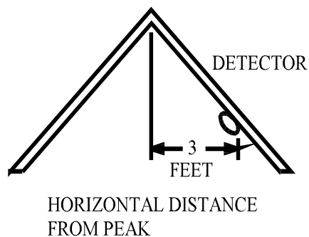
Obr. 5: DOPORUCENI PRO UMISTENI DETEKTORŮ V MISTNOSTECH S NEROVNYMI STROPY
