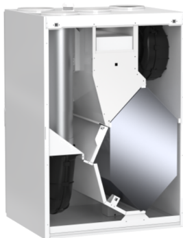
VALLOX 119 CFi
