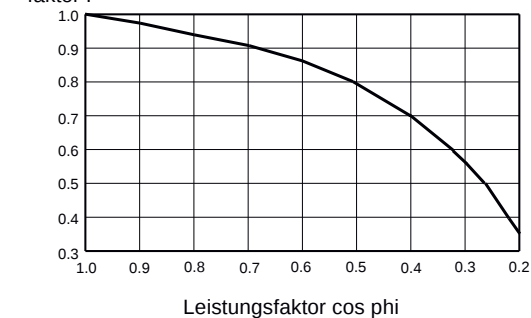
Lebensdauer-Reduktionsfaktor bei verschiedenem cos phi
