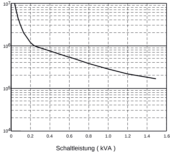
Kontaktlebensdauer für Wenderelais
