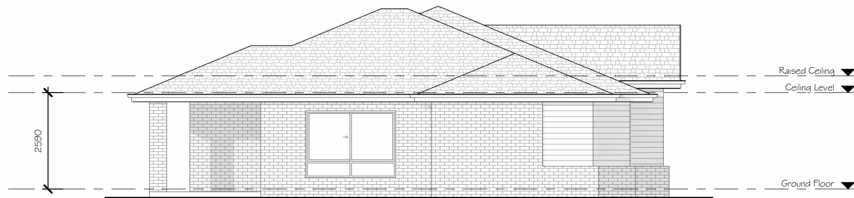
2 ELEVATION 2 1 : 100
