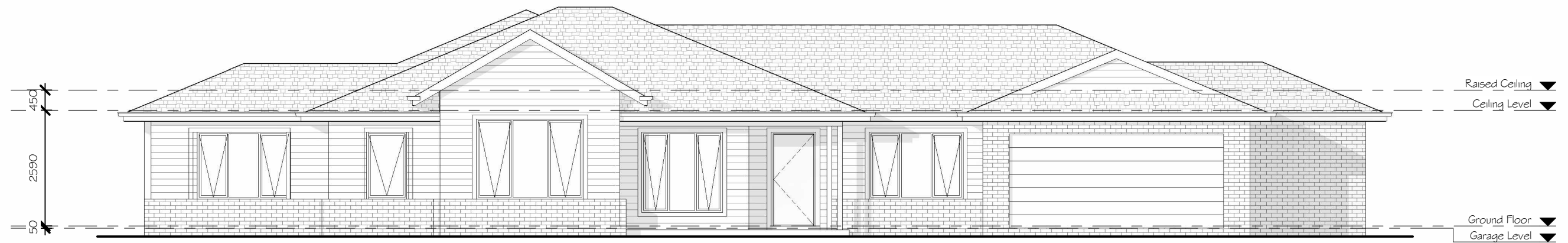
1 ELEVATION 1 1 : 100
