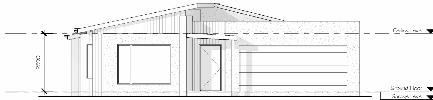
1 ELEVATION 1 1 : 100
