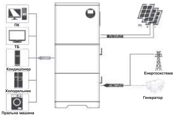
Схема системи
