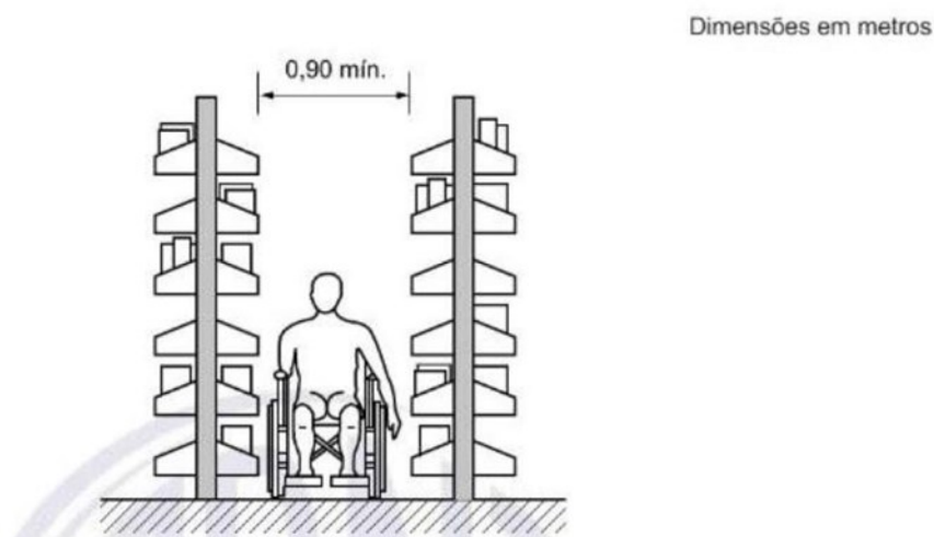
Figura 25 – Exemplo Vista Frontal do espaçamento segundo NBR 9050/2015 para as estantes da Biblioteca assegurando acessibilidade para cadeirante.
