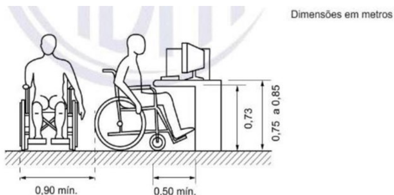
Figura 26 – Exemplo Terminais de Consulta segundo NBR 9050/2015
