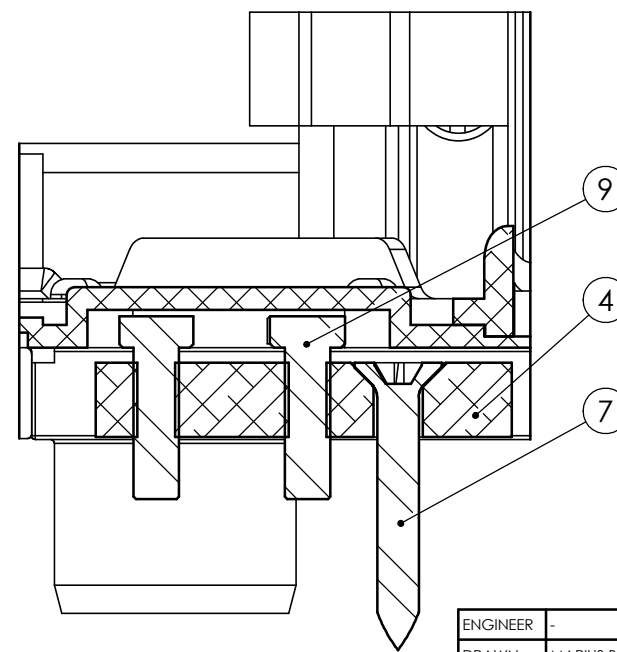
SECTION D-D
