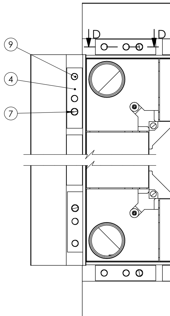
SECTION A-A
