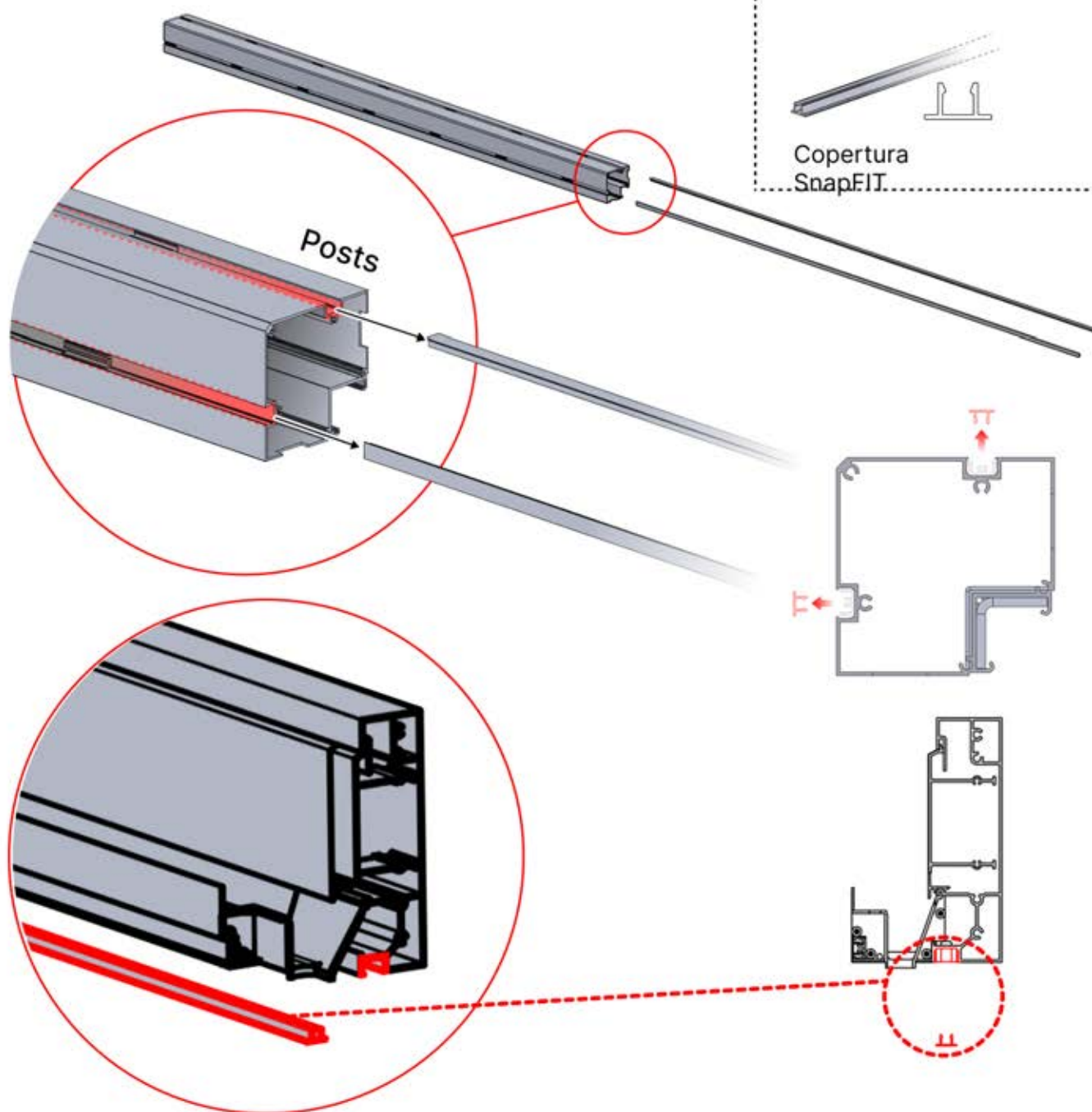
PN-200000512 clip di copertura SnapFIT
