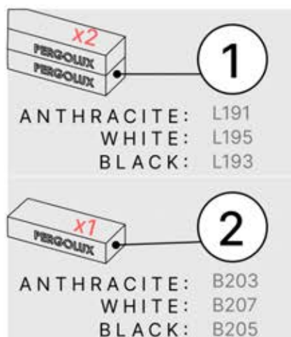
P.PERGOLA 3M FS LOUVER PN-200002714
