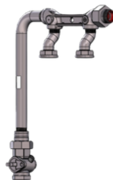
■ STANDARD METER BAR
