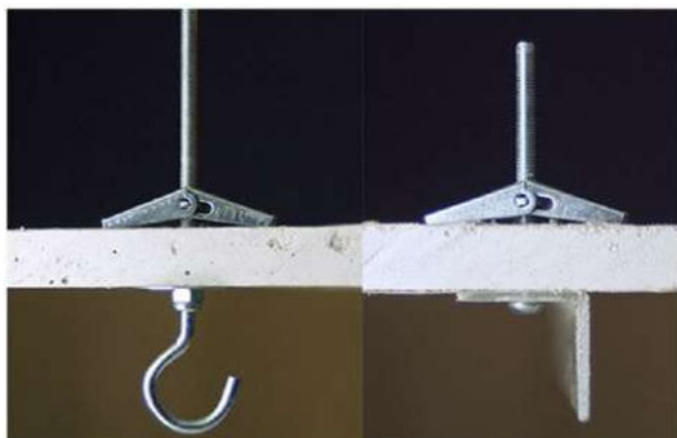
Vijak padobran sa C kukom 4x70
