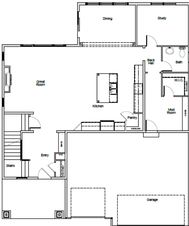
1 FIRST FLOOR PLAN A-2 SCALE: 1/8" = 1'-0"
