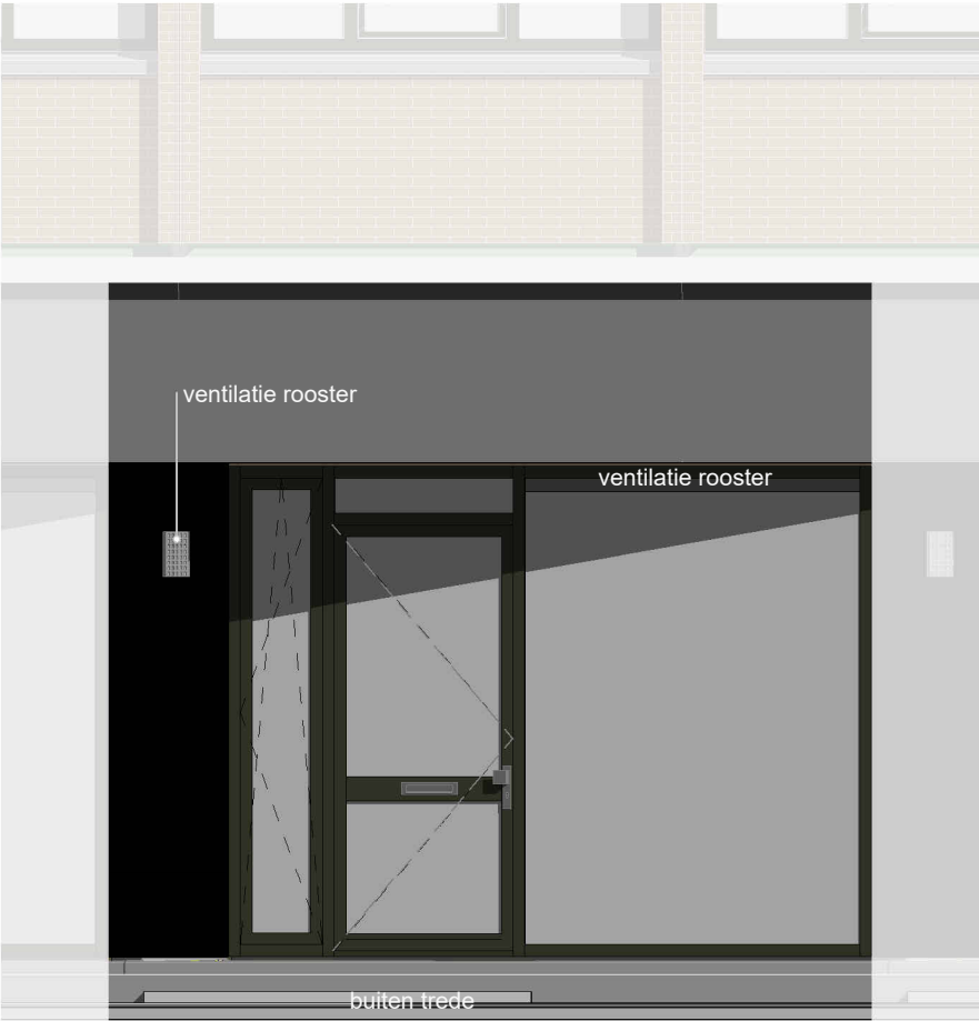
Voorgevel Loft 5- van der Rijstraat 1 : 50
