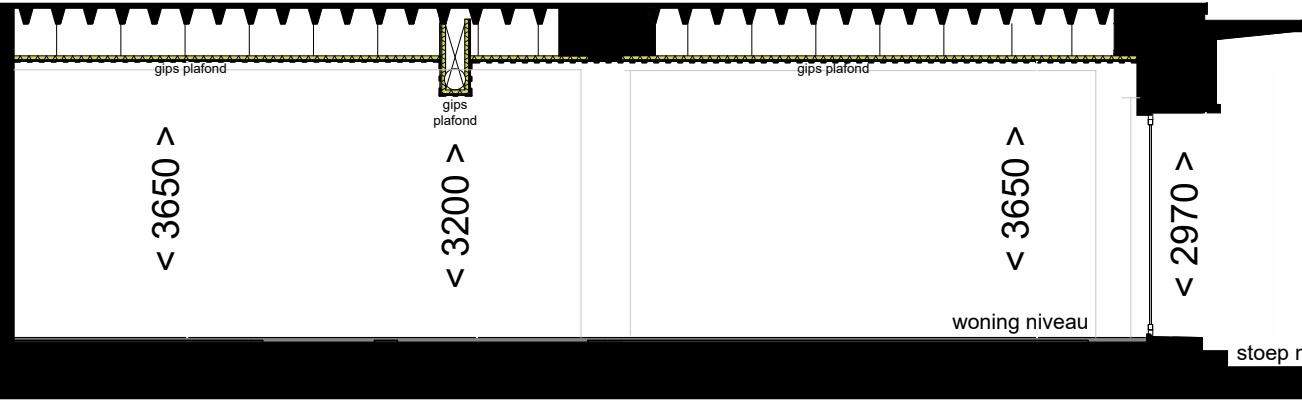
doorsnede Loft 5 1 : 100
