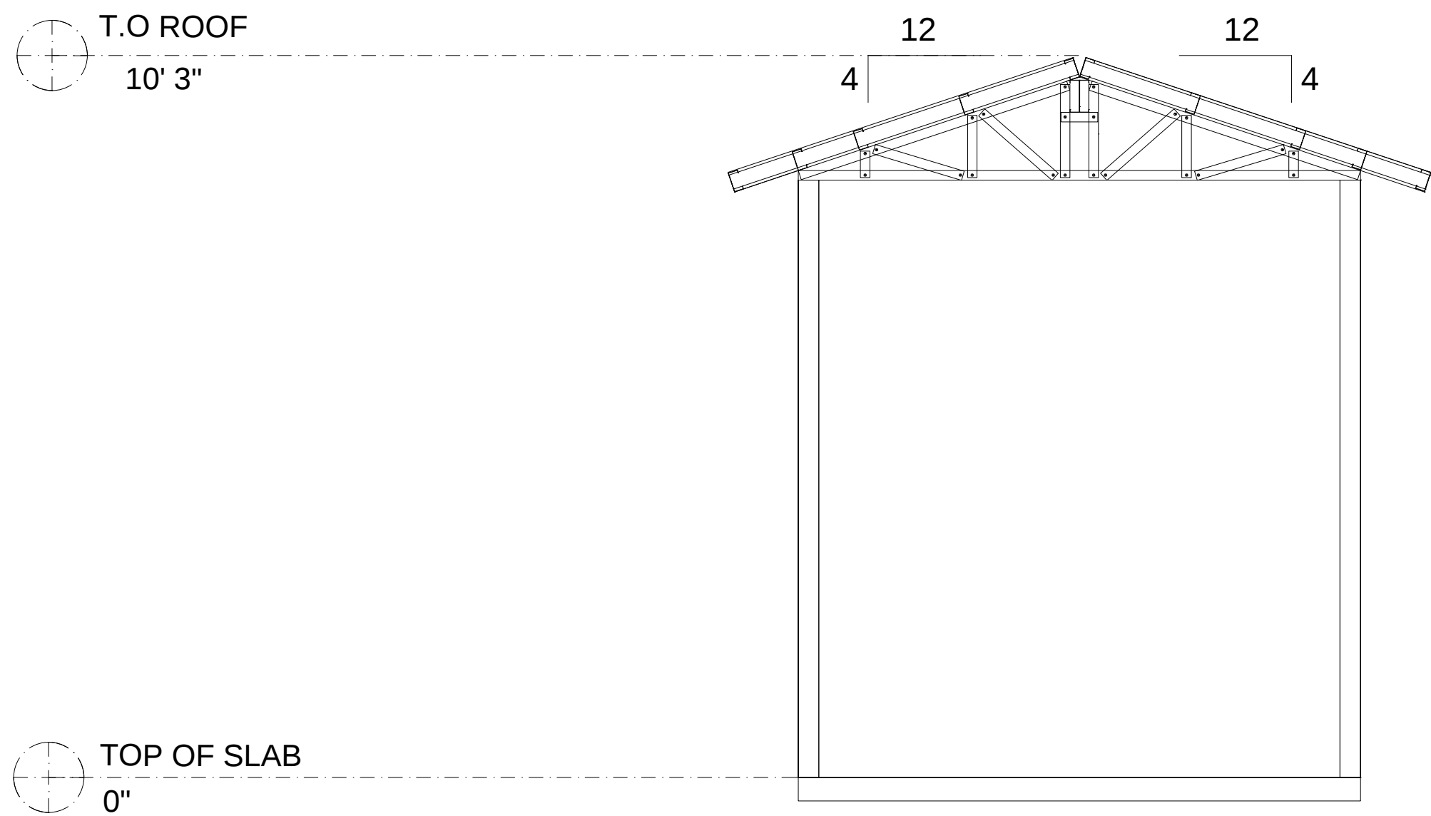
Section A-A
