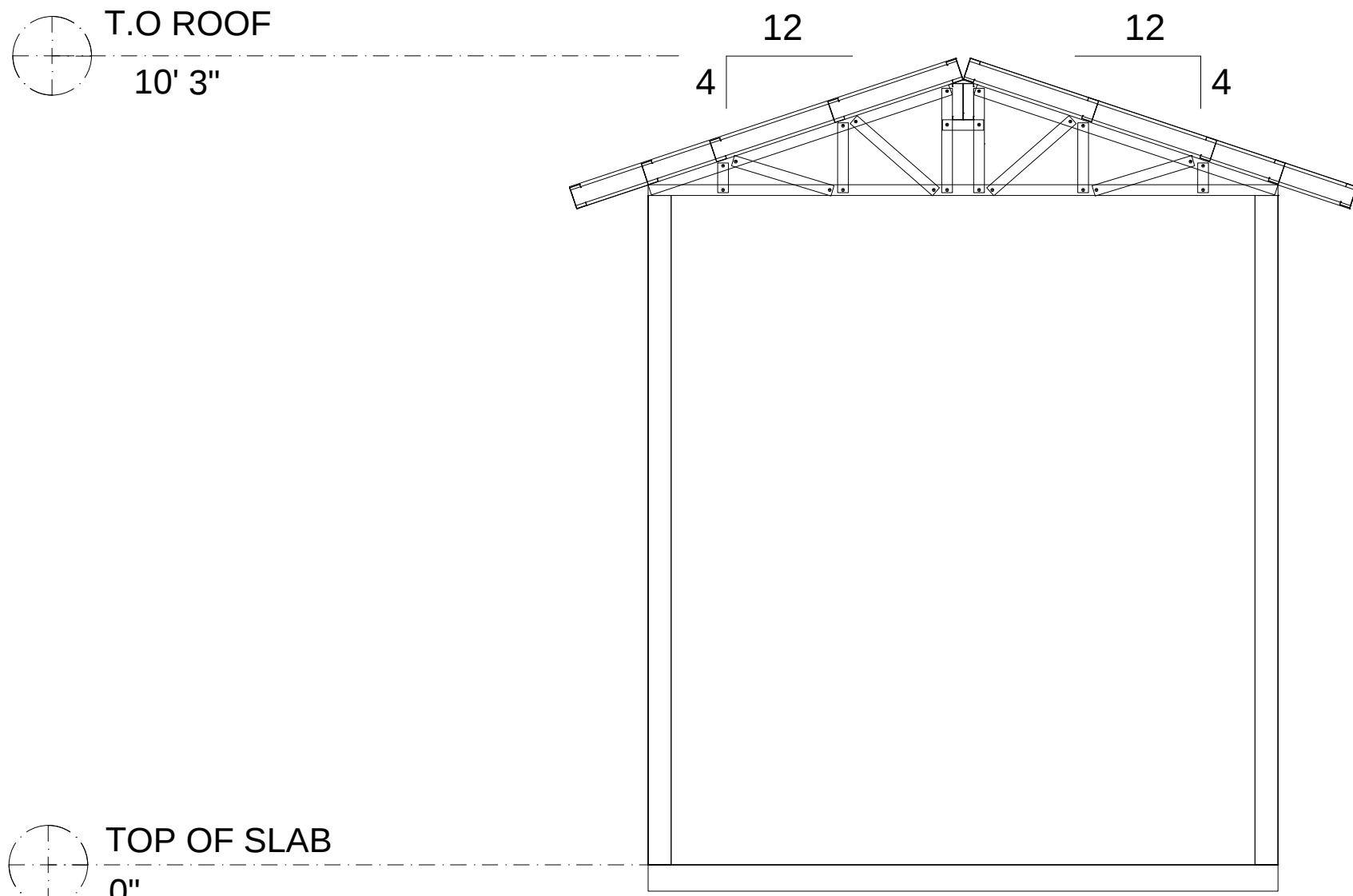
Section A-A
