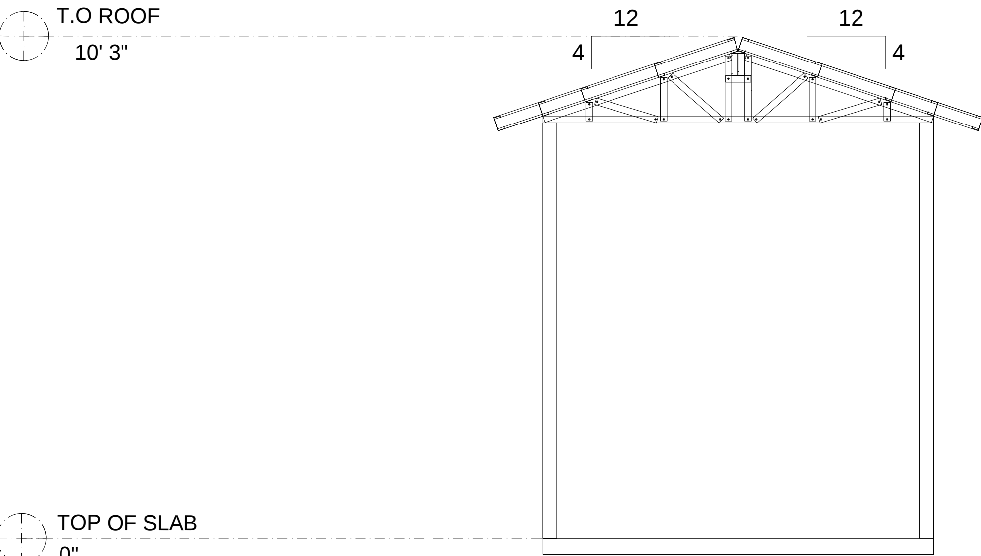
Section A-A
