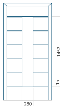
Technický výkres
