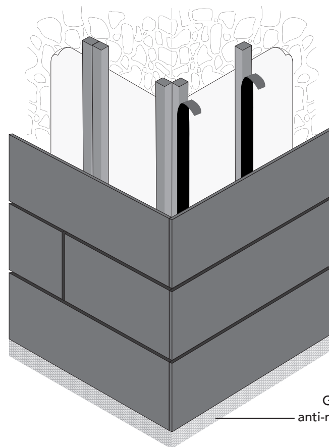
SCHÉMA DE POSE HORIZONTALE
