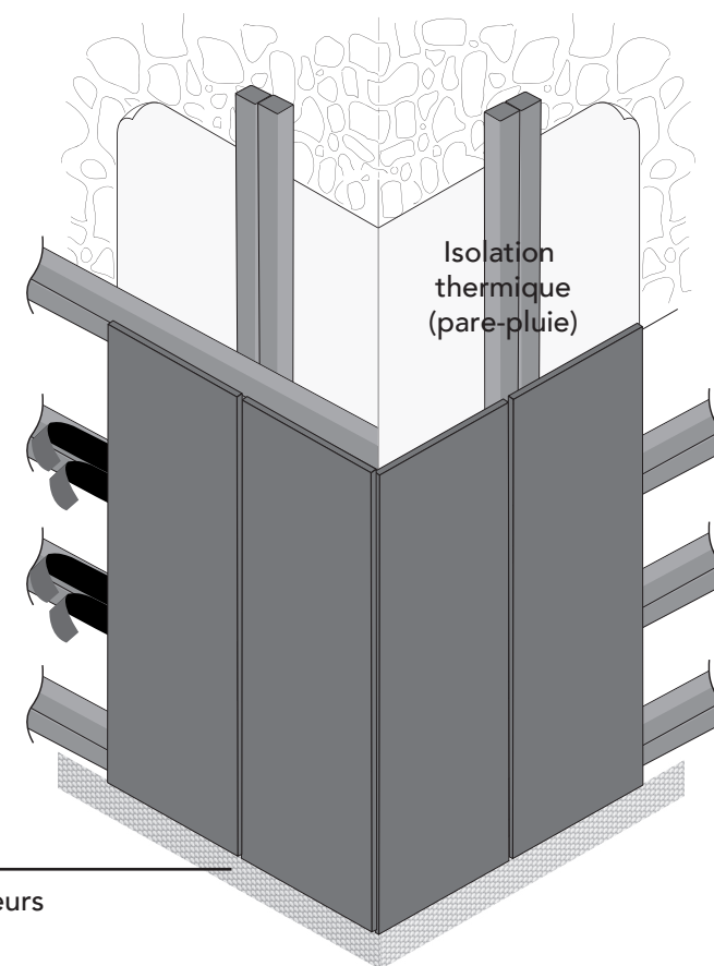
SCHÉMA DE POSE VERTICALE
