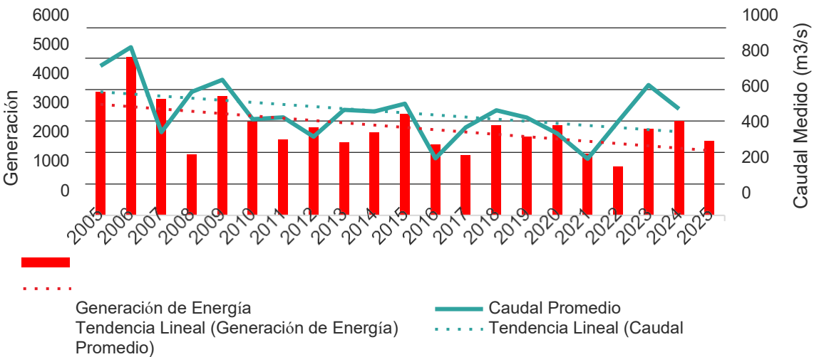
Registro de Generación Anual ARR-CH vs Recurso Hidráulico (2005–2025). Adaptado de: Generacion 93-25.xlsx Energías_crónicas_Comahue.xlsx
