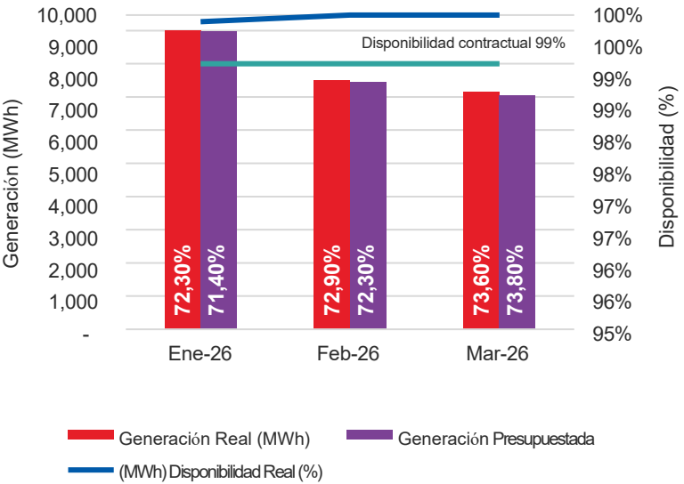
Generación Mensual de Energía (MWh) y Performance Ratio (PR): Real vs. Presupuestado. Fuente: Reporte Operaciones Parque Solar – Las Lomas Q1 - 2026
