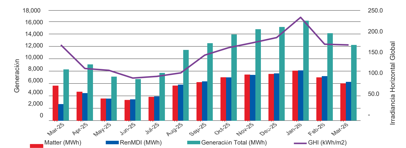
Generación mensual (MWh) desde la energización hasta marzo de 2026. Fuente: MSU Curvas de producción – GHI PVGIS.
