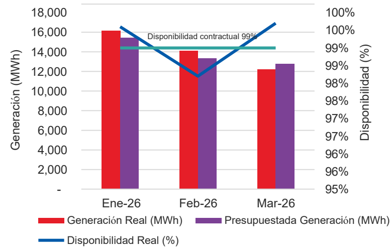
Generación Mensual de Energía (MWh) y Coeficiente de Rendimiento (PR): Real vs. Presupuestado. Fuente: Reporte Operaciones Parque Solar – Villa Angela Q1 - 2026
