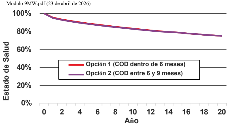
Curva de Degradación del SOH del Sistema - Planta BESS Villa Rosa. Adaptado de: Argentina MSU Matheu 150MW750MWh Proposal (0.2P-20ft HC) - 20260126.pdf BESS (20 de septiembre de 2025)
