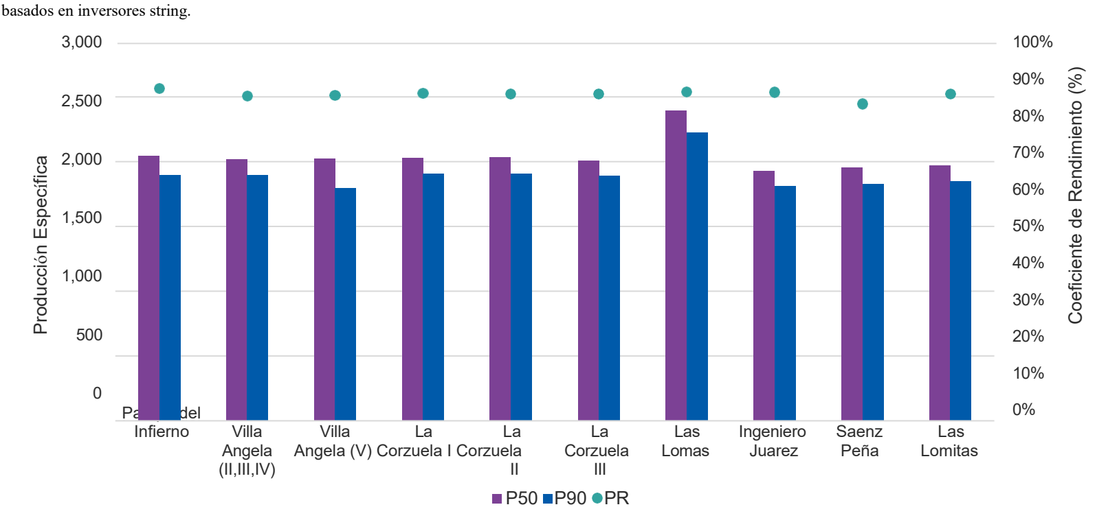
Producción Específica (kWh/kWp) – Evaluación de Producción Energética para Activos Operativos y en Desarrollo. Adaptado de: Estudio de Recurso Solar e Informes de Producción de Energía elaborados por Arengy, Enertis y MSU.
