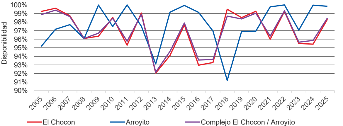
Registro de Disponibilidad Anual ARR-CH (2005–2025). Adaptado de: Disponibilidad Histórica.xlsx
