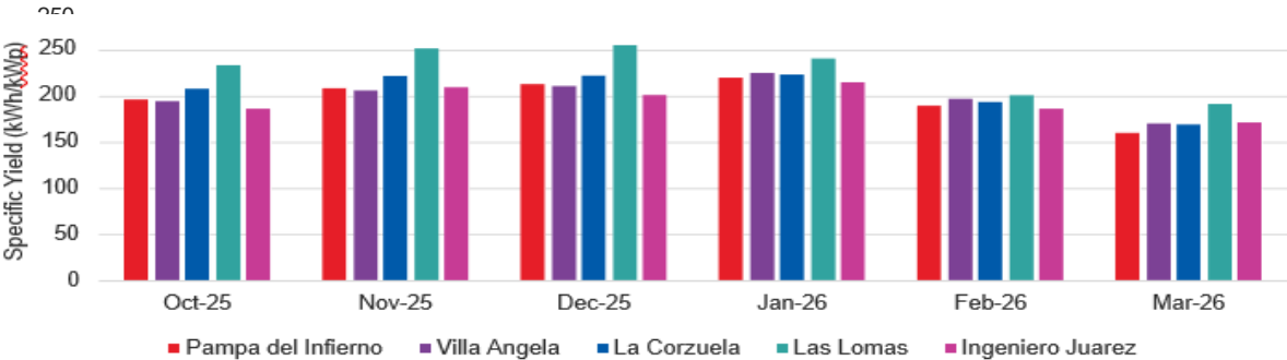
Monthly Specific Generation (kWh/kWp). Source: MSU Curvas de producción.
