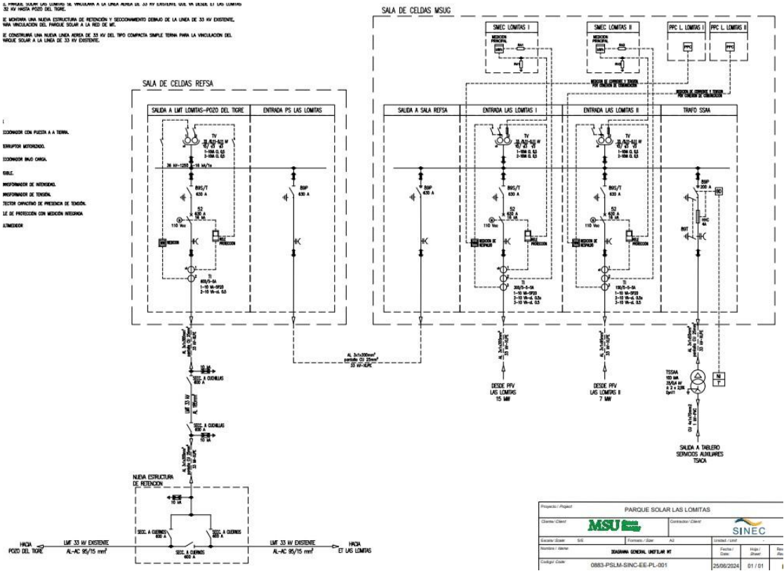
Diagrama Unifilar Las Lomitas. Fuente:0883-PSLM-SINC-EL-EE-001_E_PFV Las Lomitas - Unifilar 33 kV.pdf
