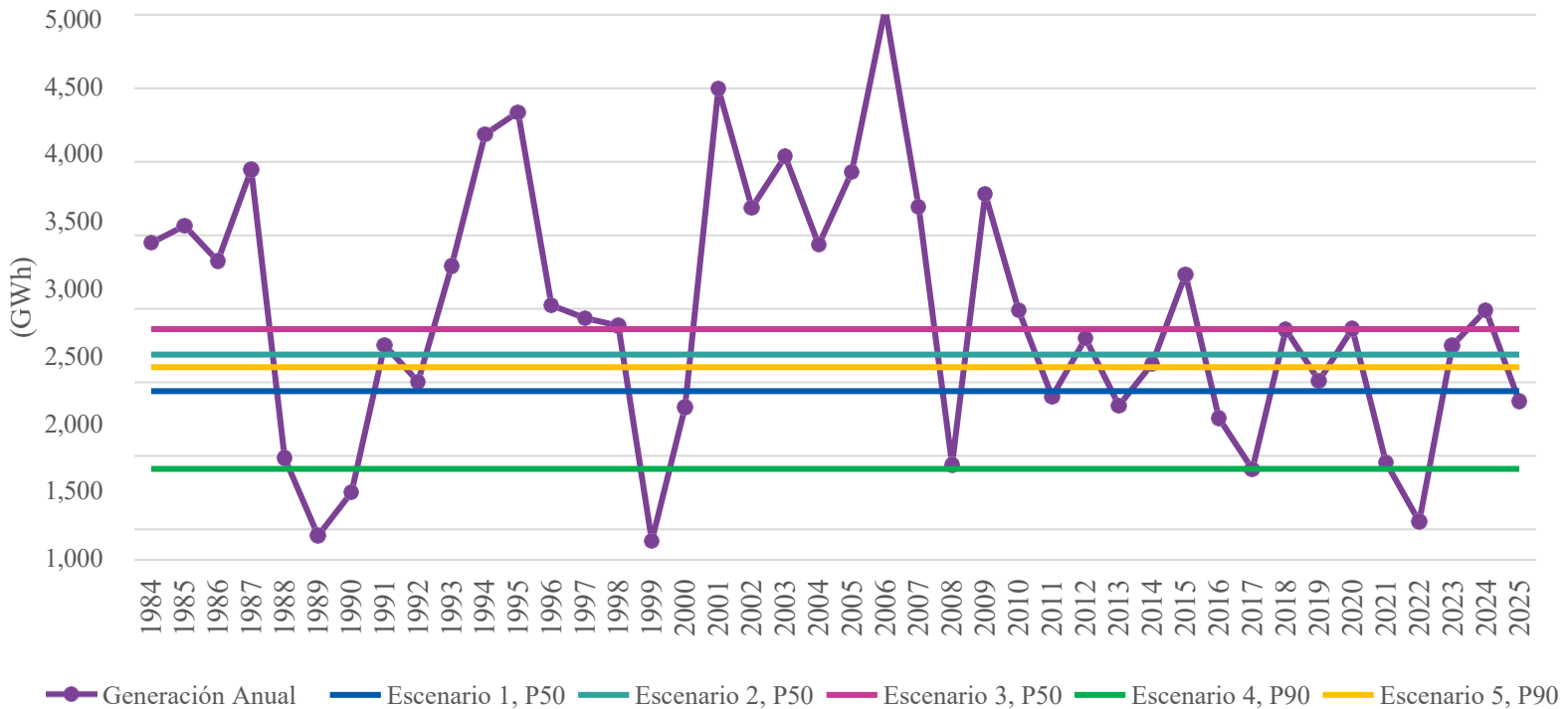
Generación histórica anual y escenarios de producción
