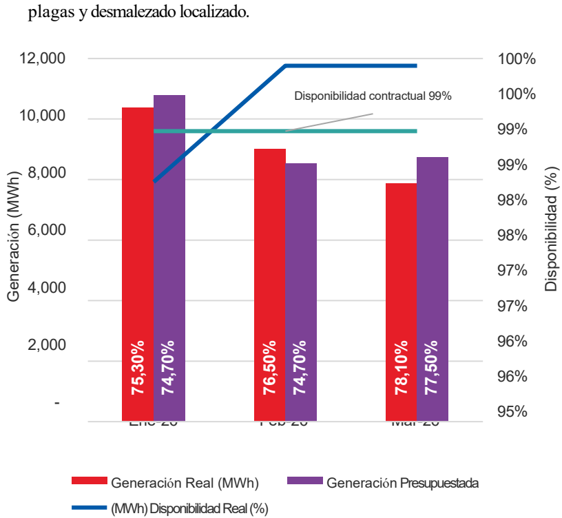
Generación Mensual de Energía (MWh) y Performance Ratio (PR): Real vs. Presupuestado. Fuente: Reporte Operaciones Parque Solar – La Corzuela Q1 - 2026
