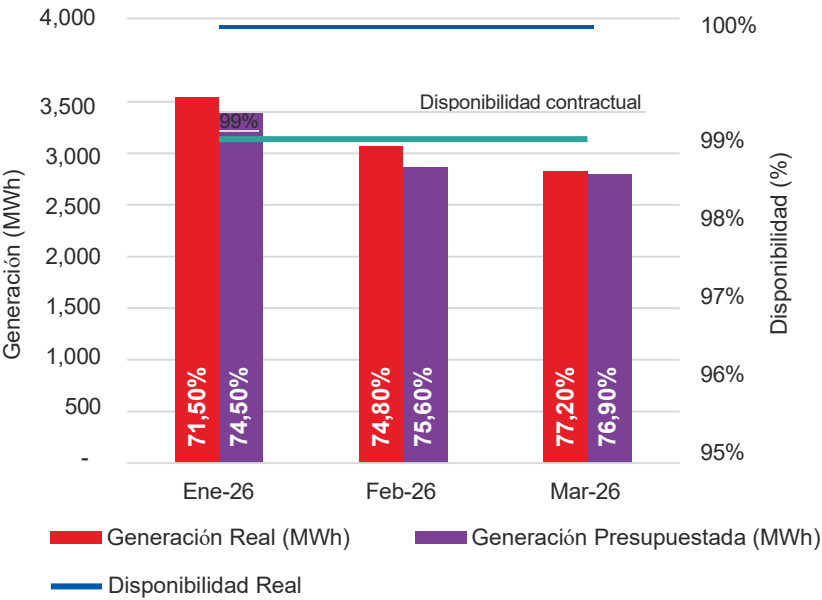
Generación Mensual de Energía (MWh) y Performance Ratio (PR): Real vs. Presupuestado. Fuente: Reporte Operaciones Parque Solar – Ingeniero Juárez Q1 - 2026
