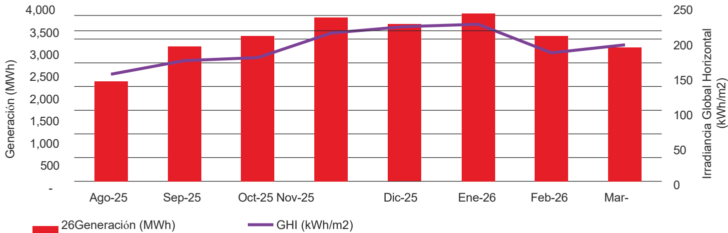
Generación mensual (MWh) desde la energización hasta marzo de 2026. Fuente: MSU Curvas de producción – GHI PVGIS.
