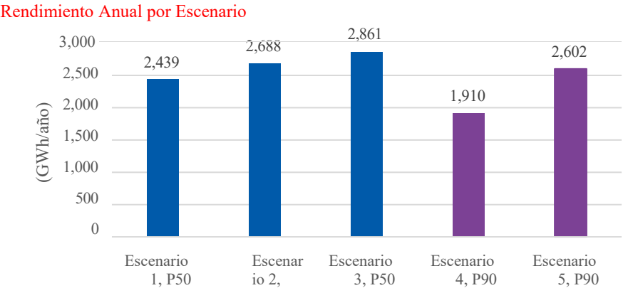
Características principales de la generación anual estimada por escenario Fuente: adaptado del archivo "P90-envío" de MSU
