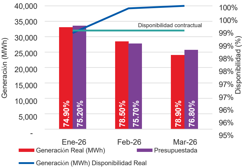
Generación Mensual de Energía (MWh) y Coeficiente de Rendimiento (PR): Real vs. Presupuestado. Fuente: Reporte Operaciones Parque Solar – Pampa del Infierno Q1 - 2026
