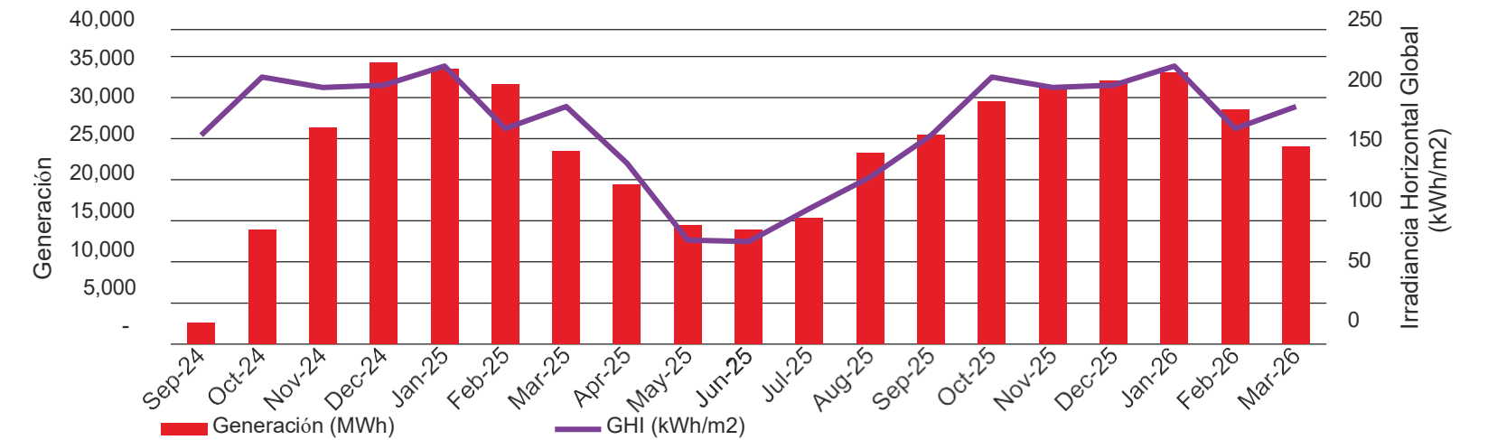
Generación mensual (MWh) desde la energización hasta marzo de 2026. Fuente: MSU Curvas de producción – GHI PVGIS.
