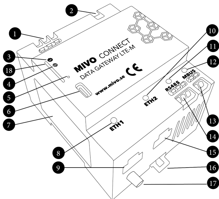
Figur 2 Produktbeskrivning
