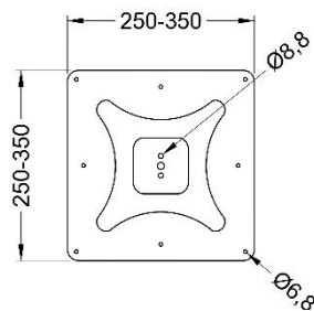
Press Plate
