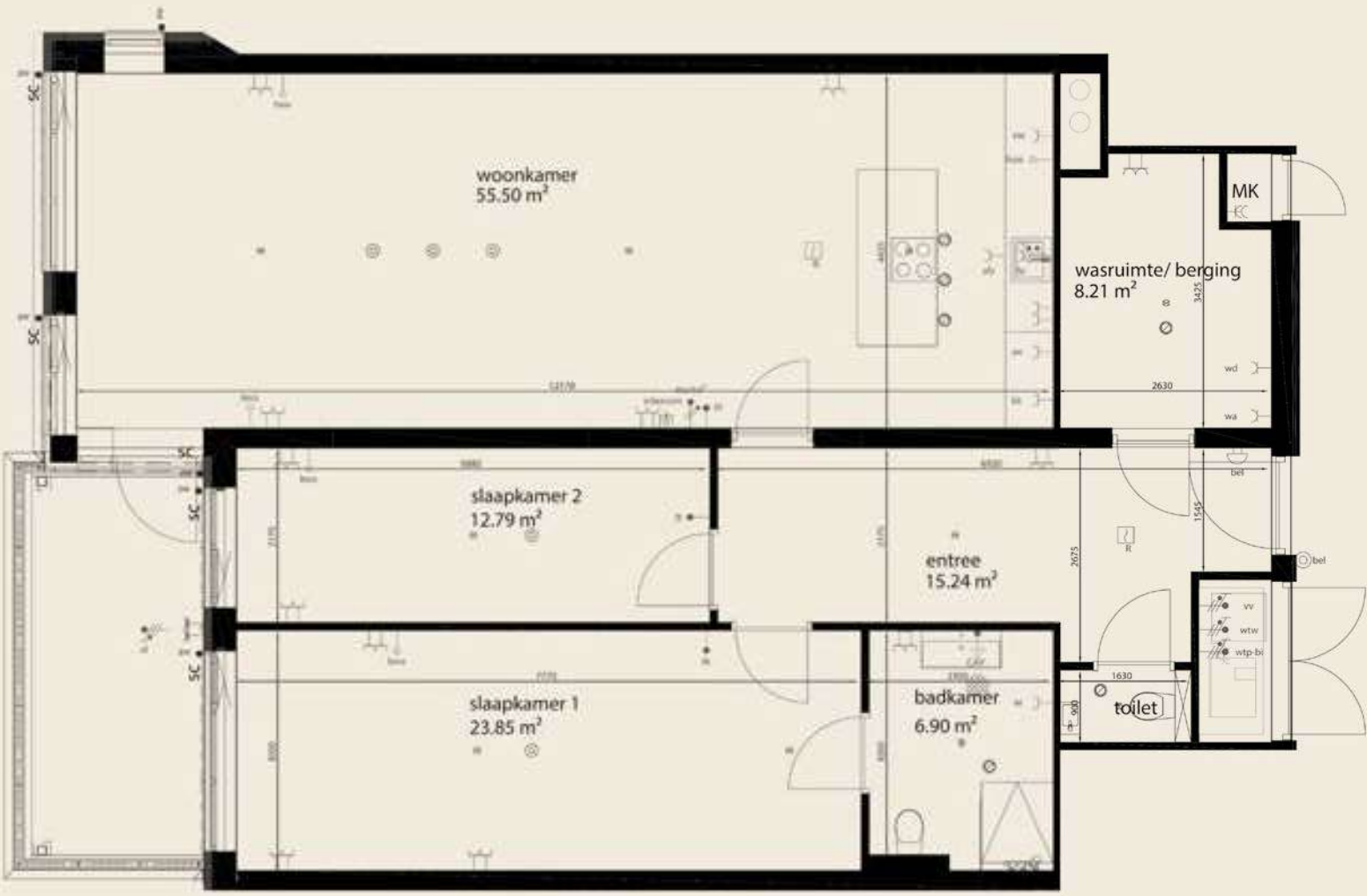
Renvooi Elektra Algemeen woning:
