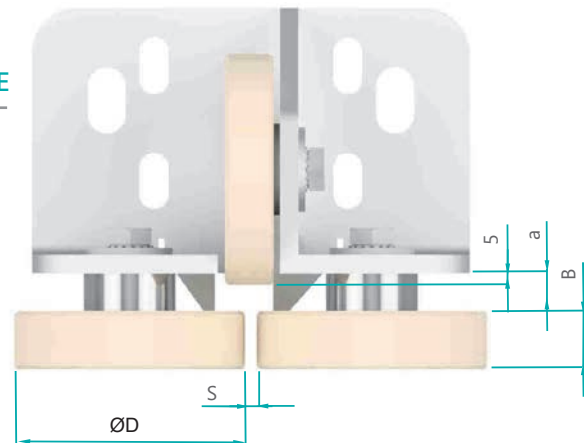
ROLLENFÜHRUNG: RFS
