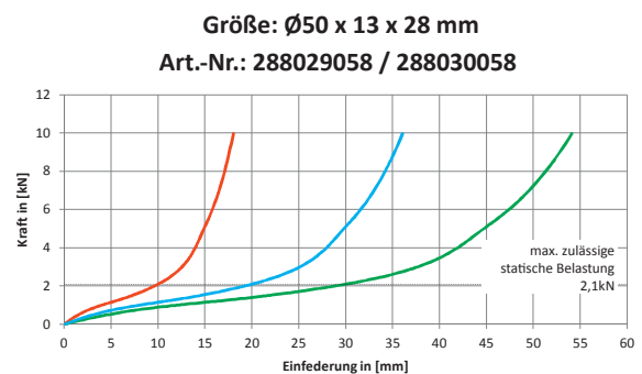
VERSION 3 – Typ A + Typ B + Typ B GRÜNE KENNLINIE
