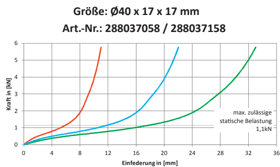
VERSION 1 – Typ A ROTE KENNLINIE
