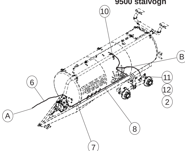
9500 stålvogn
