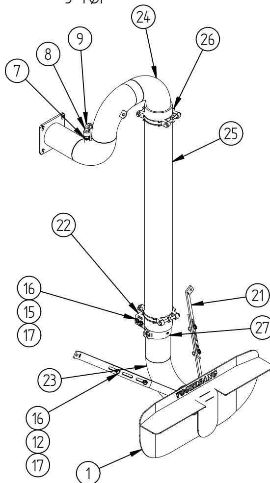
5" rør
