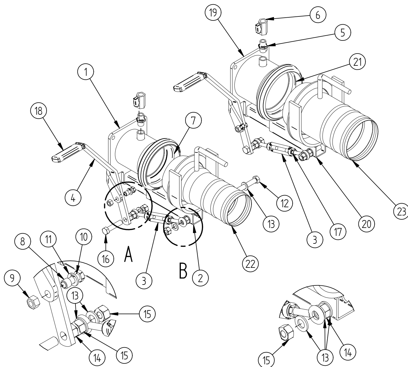
Detalj A
