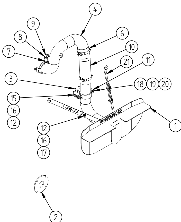
4" rør
