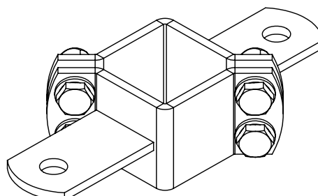
2-Veis Klammer 50x50
