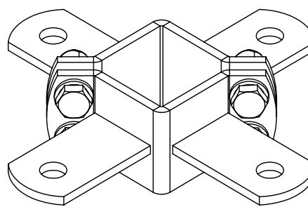
4-Veis Klammer 50x50
