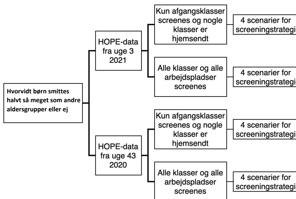
Diagram 1 Diagram over scenarietkombinationer. De fire scenarier indeholder i alt 20 kombinationer, når der varieres i compliance og test-sensitivitet.
