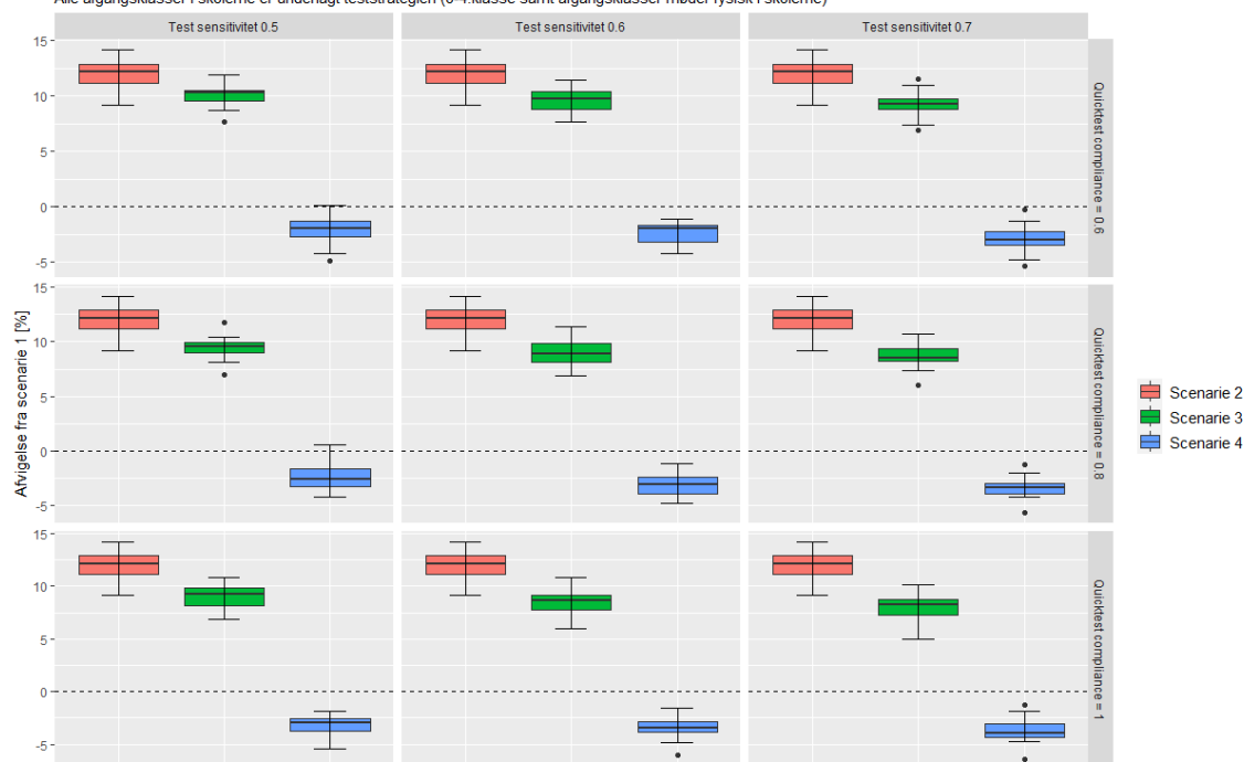
Figur 3 Kontakttal for scenarierne præsenteret i tabel 3 for alle 20 simulationer. Kontakttallene er skaleret ift. scenarie 1 (baseline).
