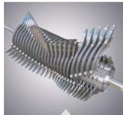
Rotor s vysokými otáčkami, velkým průměrem a možností údržby s výměnnými sekcemi prstů.
