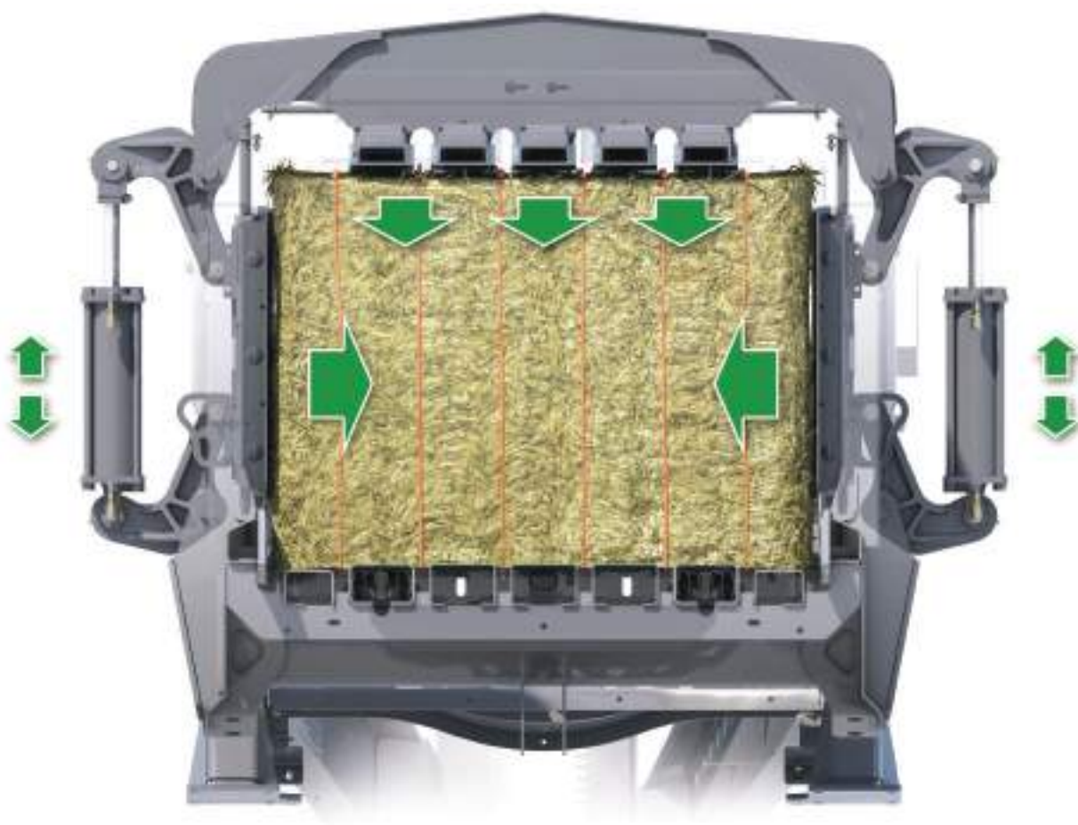
Trojcestný a dvojčinný systém pčování.
