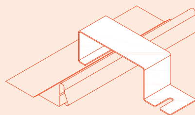
installazione di inizio posa
