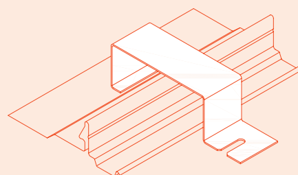
installazione di fine posa
