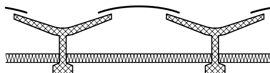
travi prefabbricate con cupolini e controsoffitto
