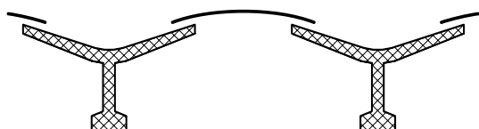
travi prefabbricate con cupolini
