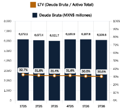
Deuda Bruta y LTV (Deuda Bruta / Activo Total) Millones de pesos y % - 1T25 a 2T26
