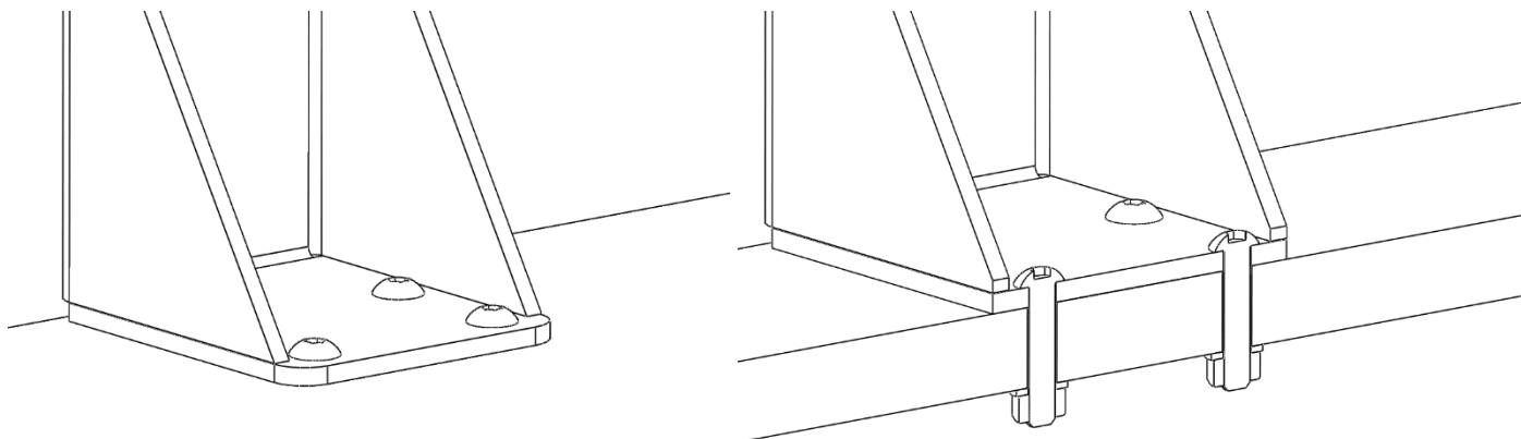
Montaje con tornillos roscados / vista de sección
